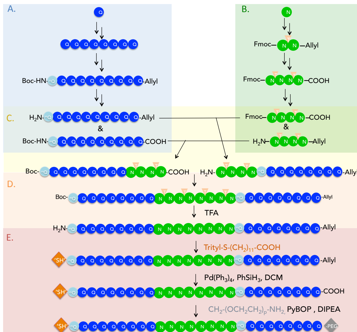
Figure 10 Schéma réactionnel de la synthèse de 'SH'-mQQ_8-N_8-mQQ_8-PEG . Les billes bleu clair, bleu foncé et vertes représentent respectivement les unités quinoléines avec une amine aliphatique, les unités quinoléines purement aromatiques et les unités naphthyridines. Les triangles orange clair représentent les groupements de protection structurale (DMB). Les fonctionnalisations des extrémités du foldamère pour des expériences de spectroscopie de force sont représentées par un carré orange pour le groupement thiol et un carré gris pour le PEG.
