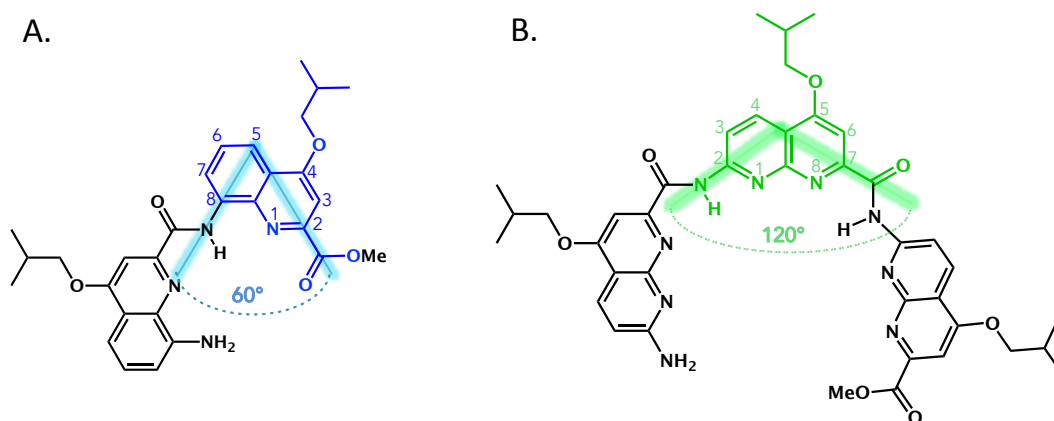
Figure 8 Structures chimiques d'un dimère de quinoléines (A) et d'un trimère de naphthyridines (B). Les angles entre les unités adjacentes sont respectivement de 60° et 120°.
