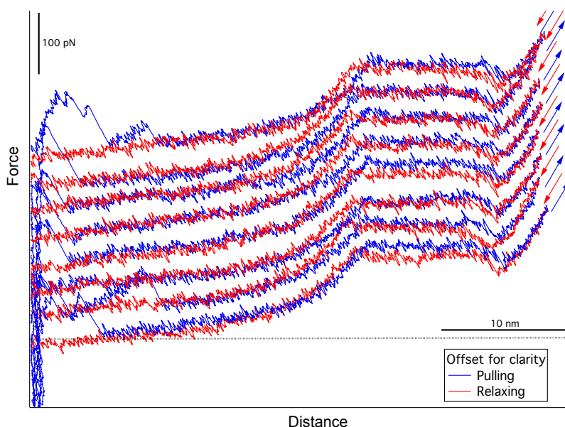
Figure 6 Série de courbes de force-distance consécutive d'expériences d'"étirement-relaxation". Les traces en bleu représentent le dépliement et les traces en rouge le signal de relaxation, chaque courbe étant décalée pour des raisons de clarté.
