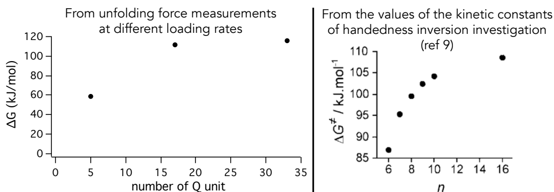
Figure 5 (A Gauche) Graphique de l'énergie libre d'une transition conformationnelle lors du dépliement forcé du foldamère, calculée à partir des forces de dépliement. (A Droite) Graphique de l'énergie libre calculées à partir des mesures cinétiques du changement du sens de l'hélicité ( n étant le nombre d'unité Q). Reproduit de la référence 9.
