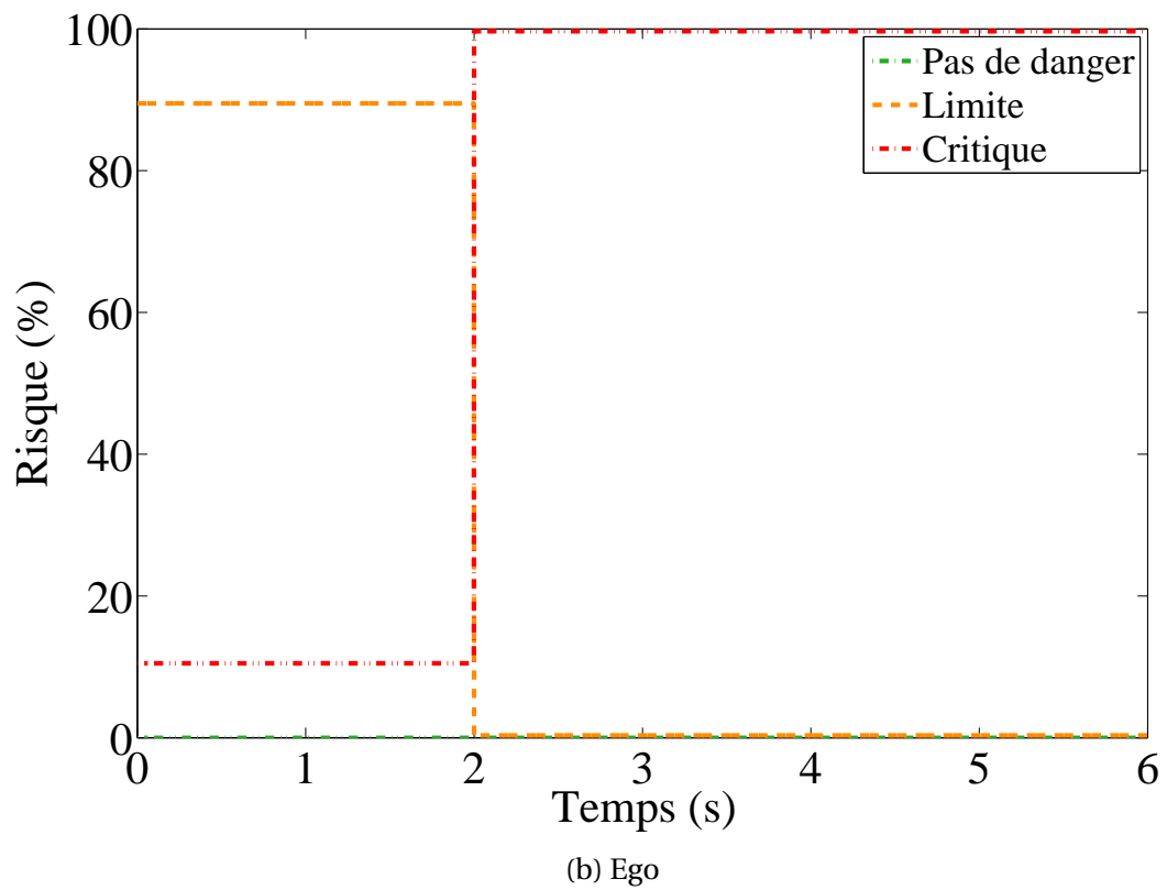
FIGURE 4.18 – Évolution du risque de Front et Ego en fonction de la communication du véhicule Obstacle
