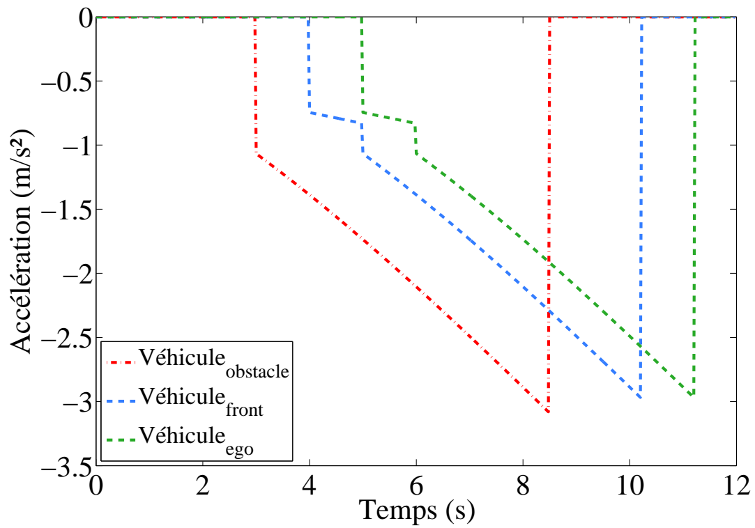
(a) Accélérations
