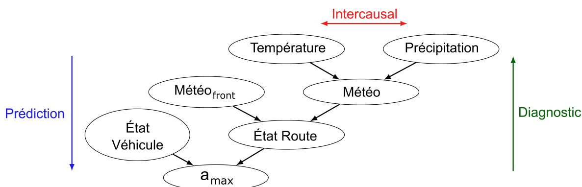
FIGURE 2.1 – Possibilité de raisonnement des réseaux Bayésiens
