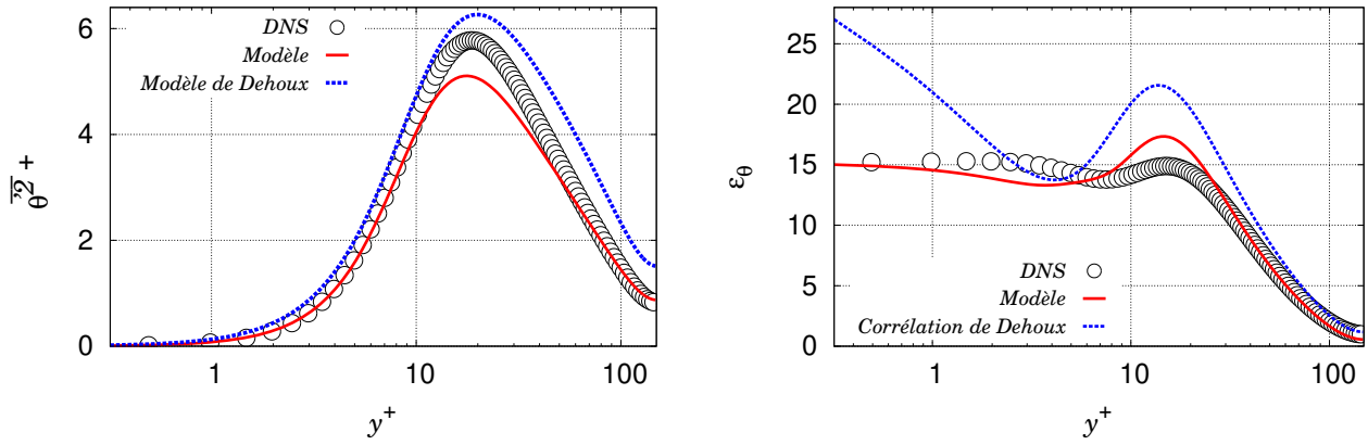
FIGURE 5.2. – Évaluation a posteriori de la variance de température \overline{\theta'^2} (gauche) et de son taux de dissipation \varepsilon_\theta (droite) pour un cas à température imposée à la paroi.
