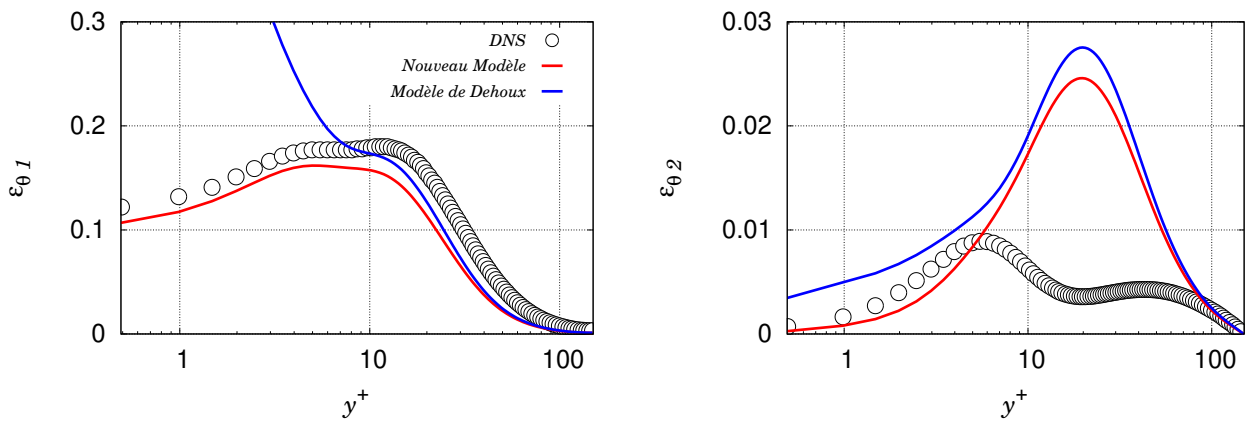
FIGURE 3.7. – Évaluation a priori du terme de dissipation \varepsilon_{\theta i} pour du transfert thermique conjugué . Gauche : composante tangentielle à la paroi; Droite : composante normale à la paroi. Données DNS d'un cas de canal plan en convection forcée de Flageul et al. (2015, 2017).
