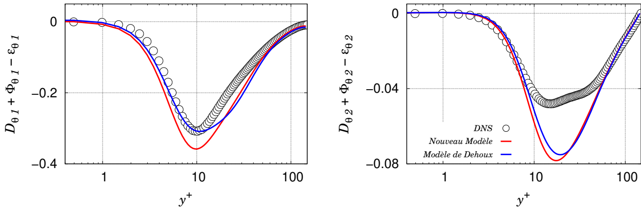
FIGURE 3.8. – Somme des termes de dissipation \epsilon_{\theta i} , de brouillage \phi_{\theta i}^* et de diffusion moléculaire D_{\theta i}^{v+\kappa} pour une température imposée à la paroi. Gauche : composante tangentielle ; Droite : composante normale à la paroi.
