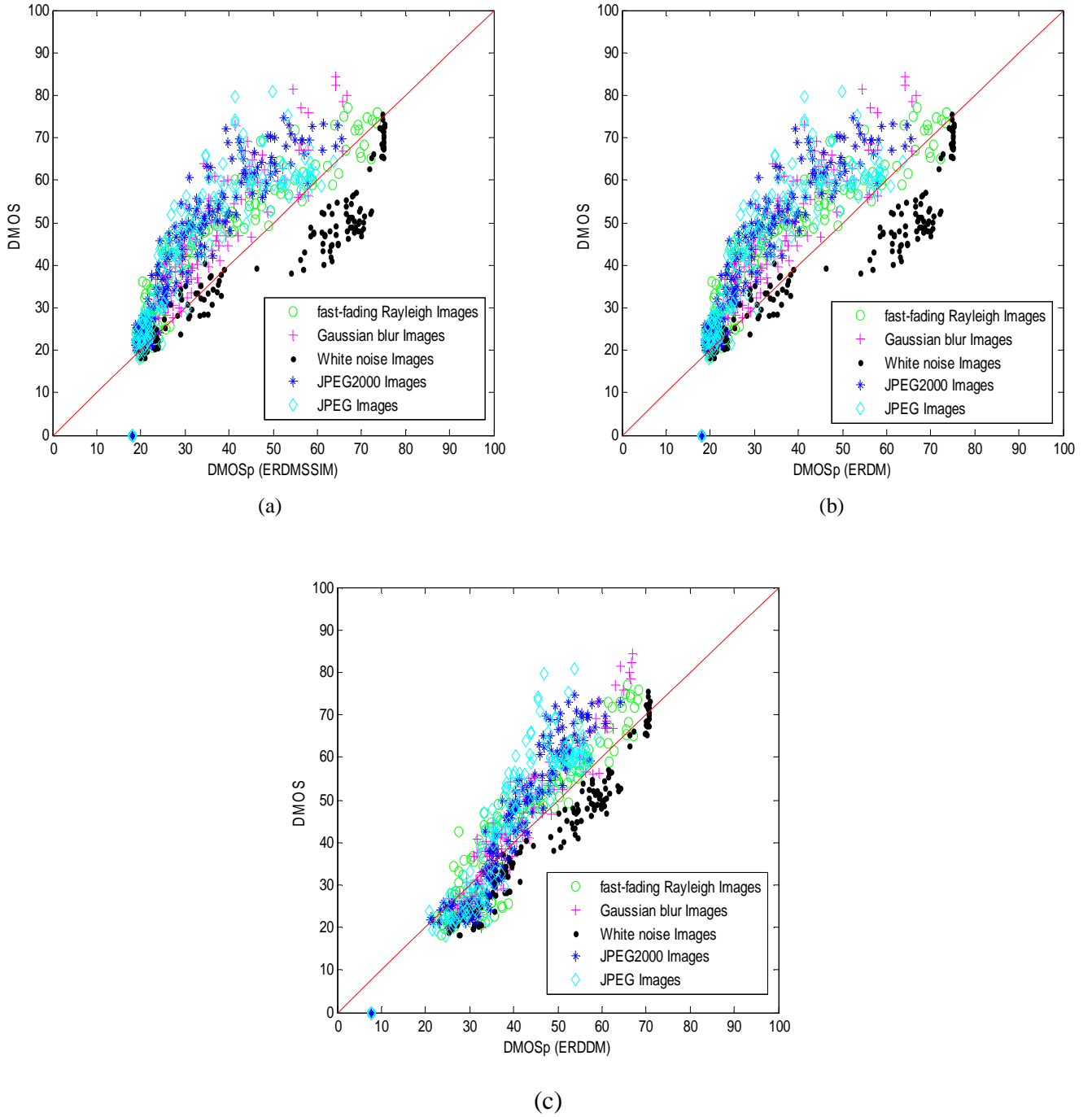
Figure 4.18: Graphe de prévisions de qualité par les six méthodes après la régression non linéaire:(a) ERDMSSIM (b) ERDM (c) ERDDM .
