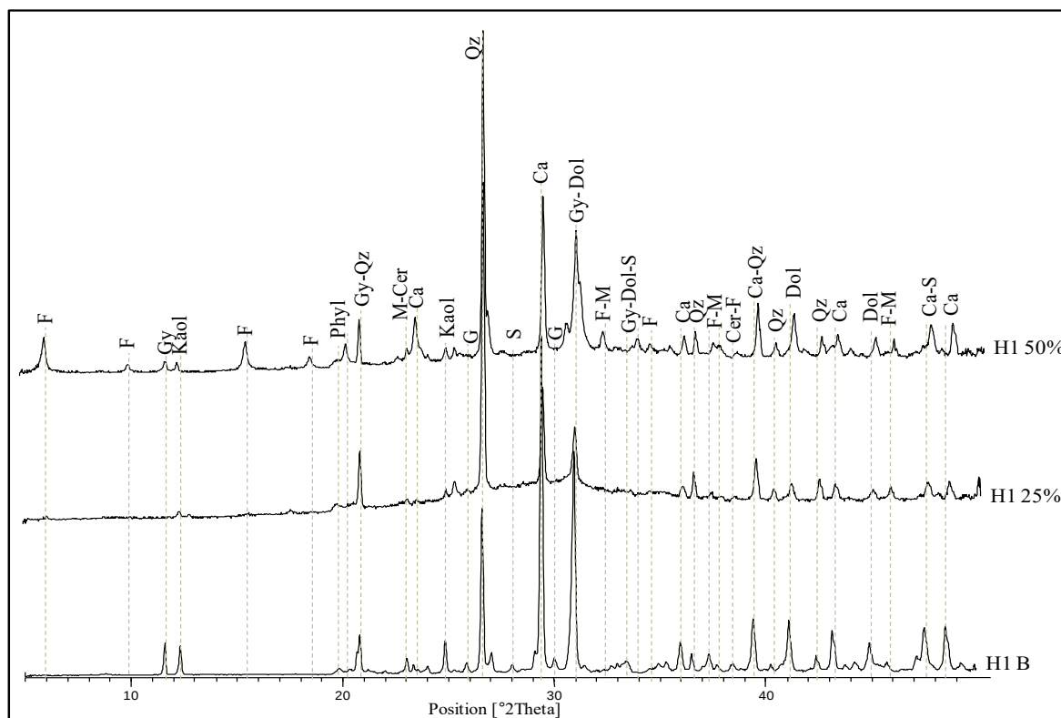
Figure 51: Comparaison des diffractogrammes des géopolymères synthétisés avec 25% et 50% de substitution par rapport à l'échantillon brut
