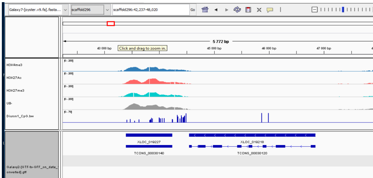
Figure 7 : Résultats du CHIP-Seq pour un échantillon sur le scaffold 296. En bleu, la marque H3K4me3, en rouge H3K27ac, en vert H3K27me3 et en gris UB- = la fraction non liée. Les pics représentent les zones enrichies du gène ou les histones possèdent les différentes marques. La hauteur des pics représente la couverture en reads. La cinquième piste correspond à la méthylation du gène, chaque barre est une cytosine méthylée, la hauteur des barres correspond au pourcentage de méthylation. En bas, le transcriptome de C. gigas a été rajouté.
