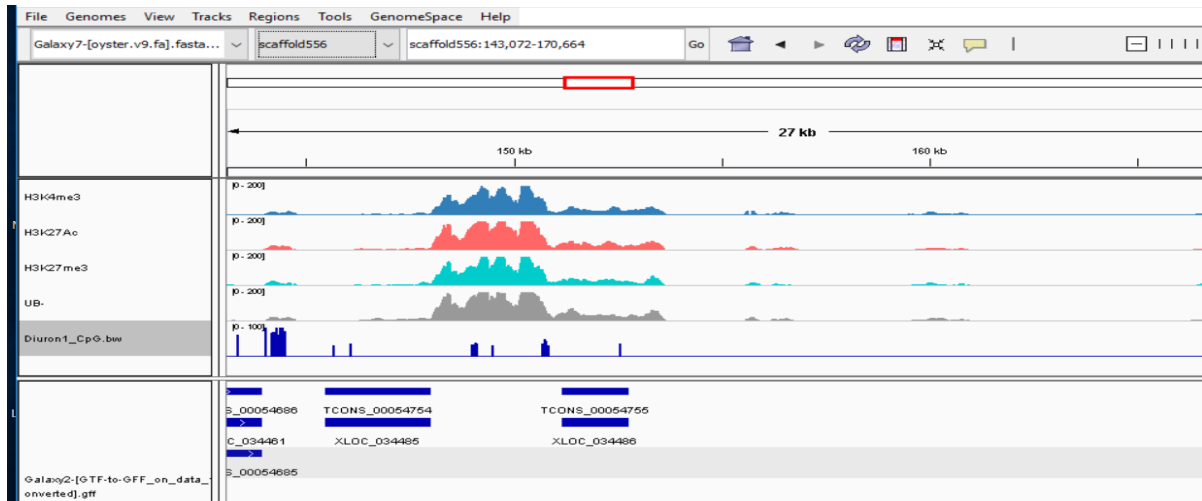
Figure 8 : Résultats du ChIP-Seq pour un échantillon sur le scaffold 556. En bleu, la marque H3K4me3, en rouge H3K27ac, en vert H3K27me3 et en gris UB- = la fraction non liée. Les pics représentent les zones enrichies du gène ou les histones possèdent les différentes marques. La hauteur des pics représente la couverture en reads. La cinquième piste correspond à la méthylation du gène, chaque barre est une cytosine méthylée, la hauteur des barres correspond au pourcentage de méthylation. En bas, le transcriptome de C. gigas a été rajouté.
