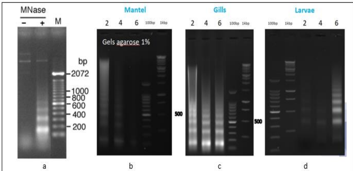
Figure 2 : Digestion à la micrococcale nucléase. a) Echelle attendue suite à une digestion à la micrococcale nucléase, les bandes blanches représentent les mononucléosomes, les dinucléosomes.... Plus la micrococcale nucléase agit longtemps plus l'ADN est dégradé et donc plus on obtient de mononucléosomes. Si la digestion n'est pas totale, nous observons différentes bandes correspondant à des mono, des di, des tri... nucléosomes. Pour le bon fonctionnement du CHIP nous devons avoir différentes taille de nucléosomes et donc observer un motif « en échelle » après la migration à l'électrophorèse. Figure tirée de (Suka et al., 2006) b) c) et d) Nos résultats de digestion pour différents tissus d'huitre (b : manteau, c : branchies, d : larves) les chiffres en haut représentent les temps de digestion en minutes (2, 4 et 6 min). 100bp et 1Kp représentent les marqueurs de tailles
