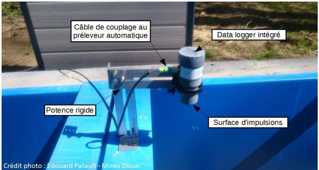
Fig. 75 : Débitmètre à ultrasons LNU300-X de la marque JJINUS.
