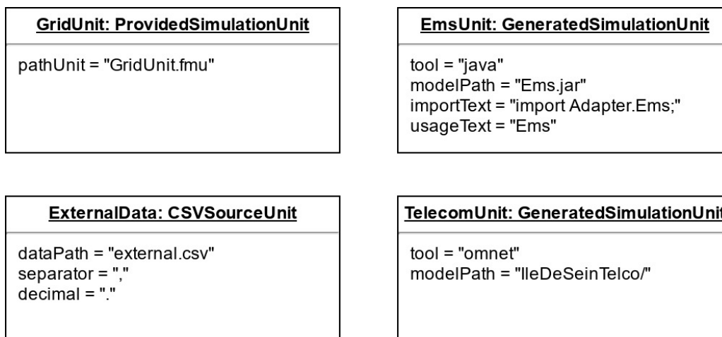
FIGURE 8.2 – SimulationUnit instanciées dans le modèle CatalogML
