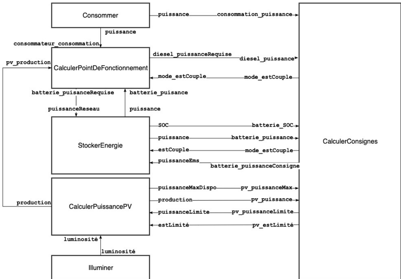
FIGURE 8.1 – Connection entre les Fonction du modèle SGridML de l'île de Sein
