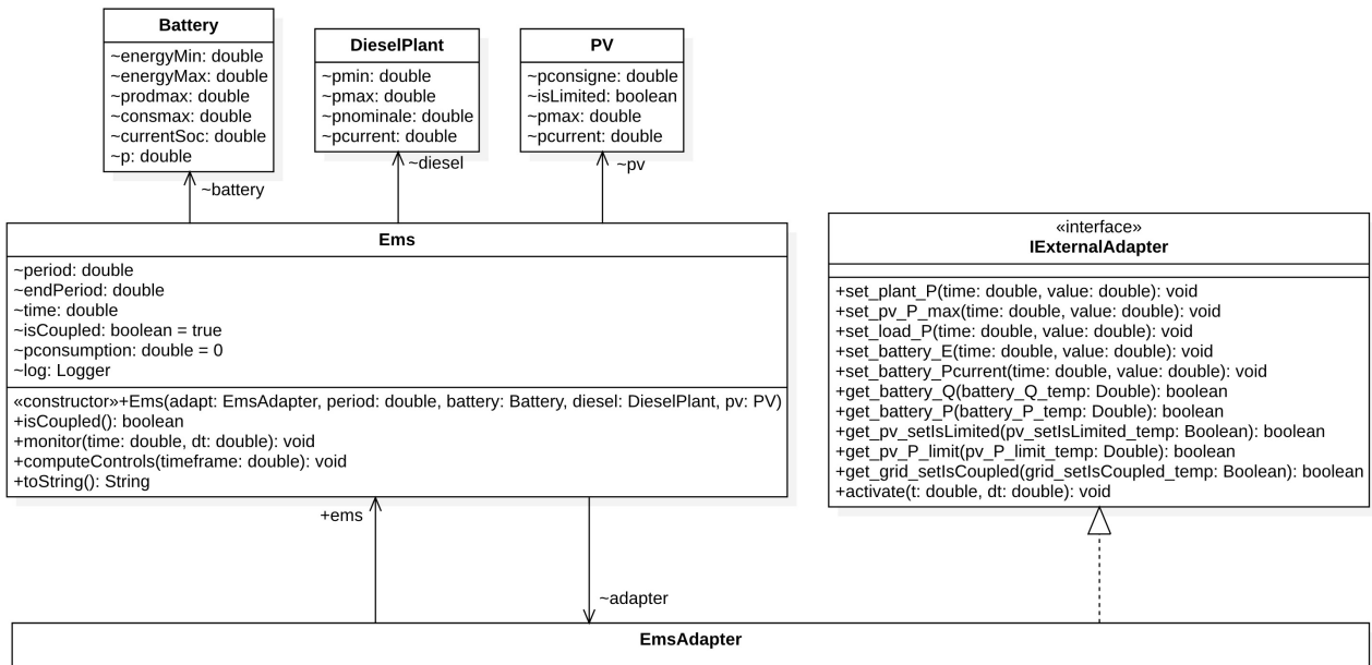
FIGURE 8.6 – Diagramme des classes Java du modèle de EMSUnit
