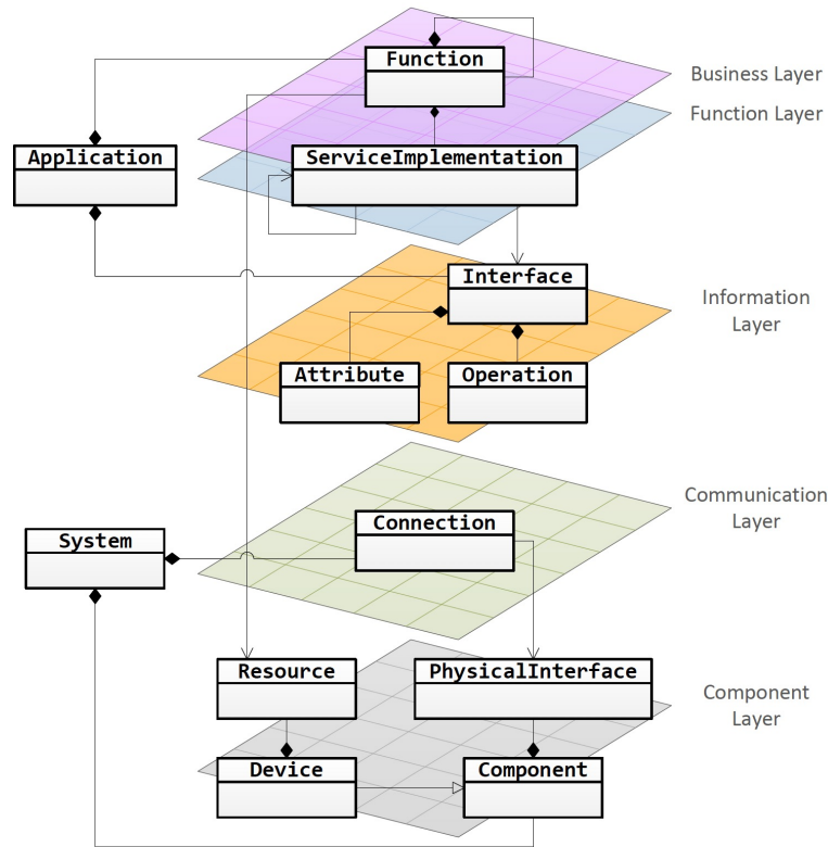
FIGURE 3.9 – Représentation simplifiée en UML des concepts du Power System Automation Language (PSAL). Source : [Andr en et al., 2017]
