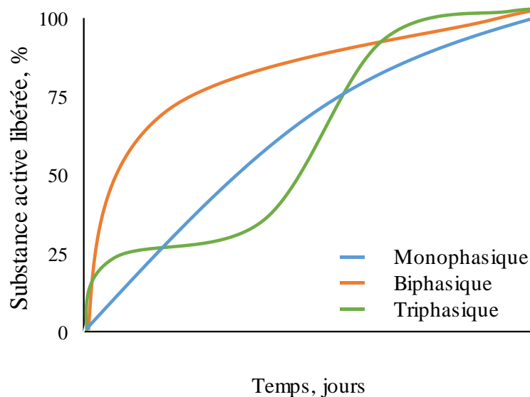
Figure 10: Représentation schématique des différents profils de libération d'une substance active à partir de microparticules.
