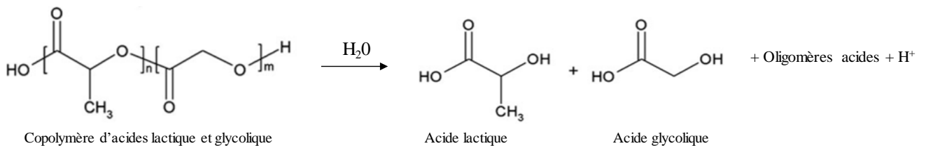
Figure 3: Réaction de dégradation du copolymère d'acides lactique et glycolique.
