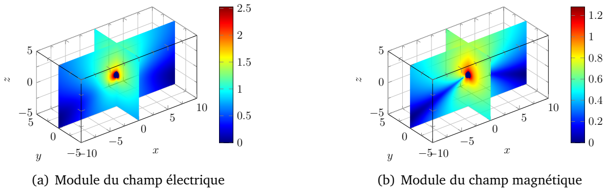
FIGURE 5.12 – Représentation du module des composantes des champs électromagnétiques diffractés en échelle logarithmique.
