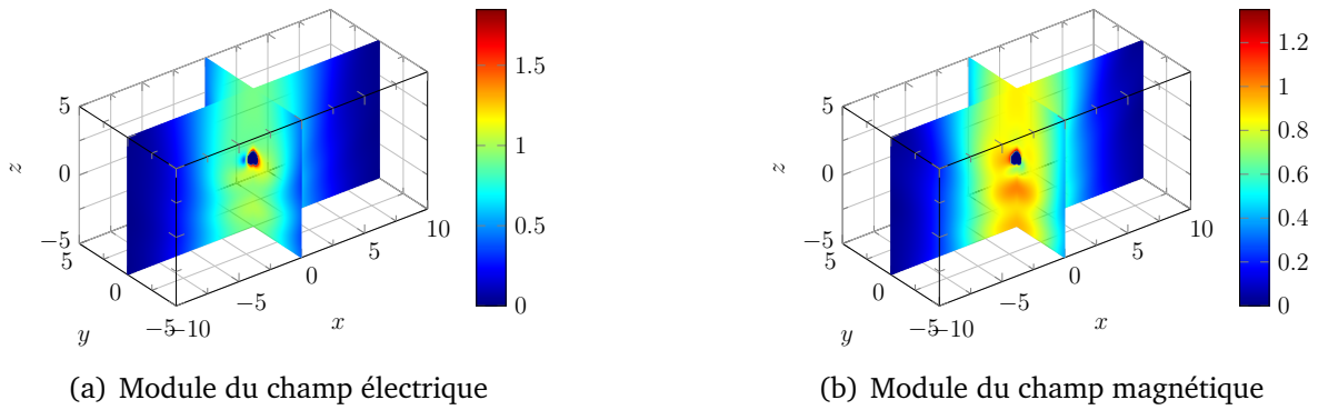
FIGURE 5.11 – Représentation du module des champs électromagnétiques totaux.
