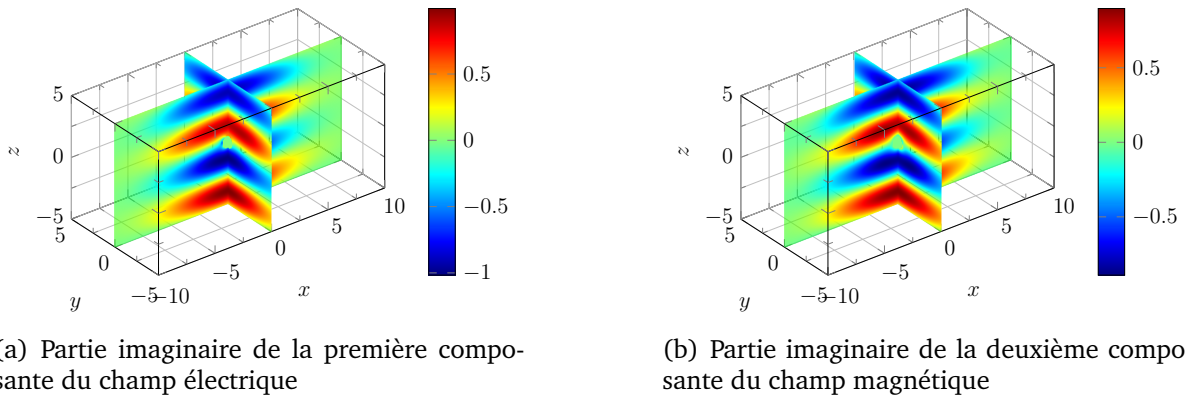
FIGURE 5.10 – Représentation de la partie imaginaire de l’une des champs électromagnétiques totaux.
