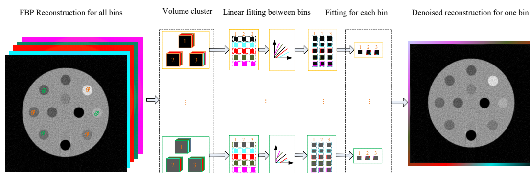
Figure 13 Cadre de la méthode proposée: débruitage de reconstruction pour une bande d'énergie.
