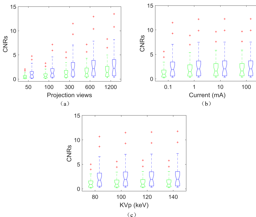
Figure 5 Comparaison entre le CT classique et l'aCT en termes de CNRs pour: (a) différents angles de projection; (b) différents courants de source; (c) différentes tensions de source.
