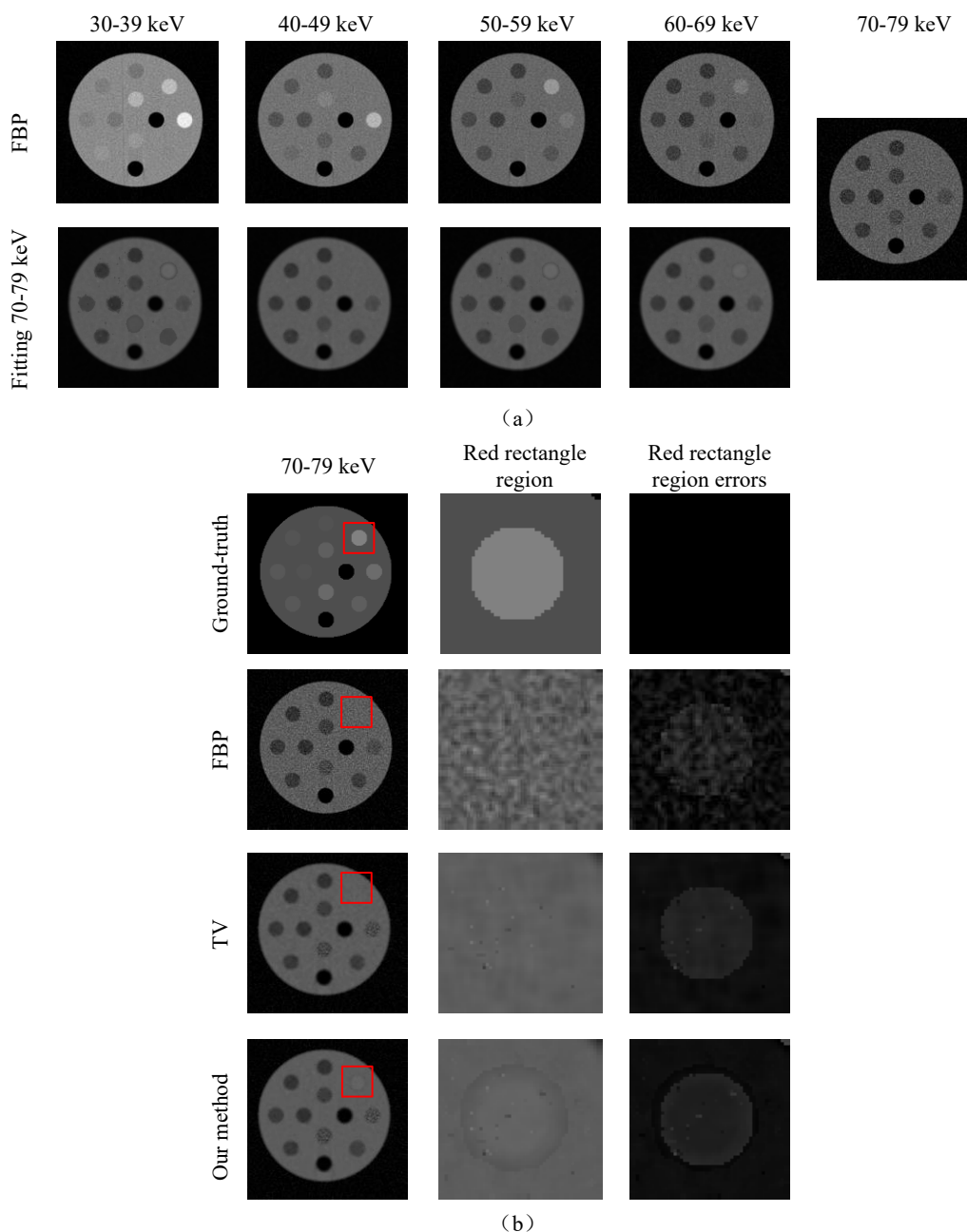
Figure 14 Comparaison de la reconstruction pour une bande d'énergie de 70-79 keV.
