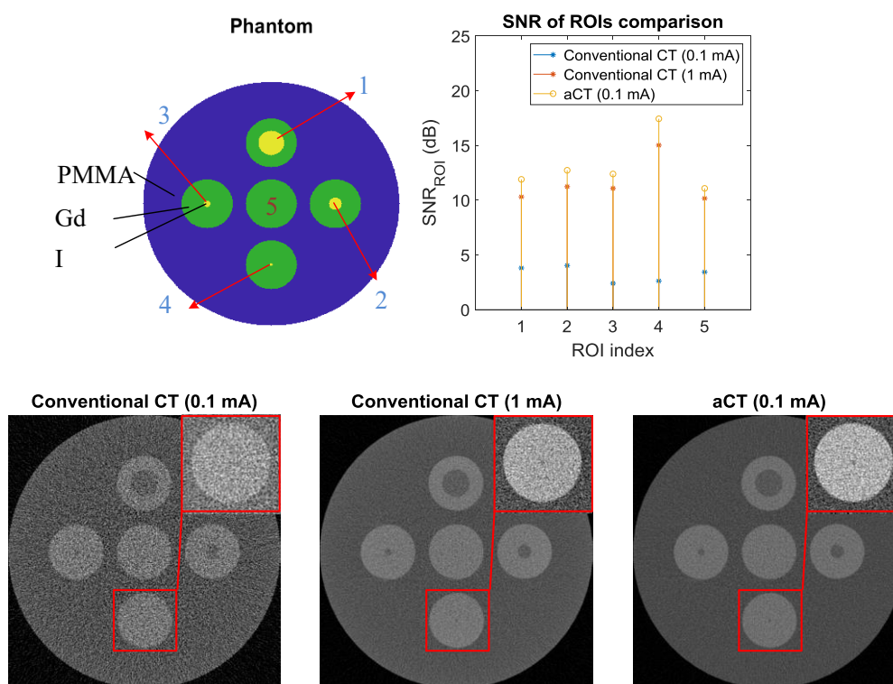
Figure 12 Comparaison entre l'image aCT du sCT et l'image CT classique. La région zoomée contient le petit trou de 3 mm de rayon (au centre de la région rempli d'iode de densité 5 mg/cc).
