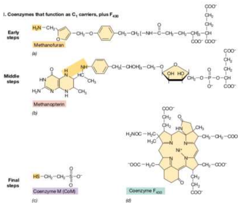
Figure 46 : Coenzymes transporteurs du carbone 1 et le coenzyme \text{F}_{430} impliqués dans la méthanogénèse (Madigan et al 2010).
