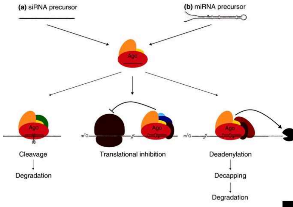
Figure 18: Modes d'action de protéines argonautes guidées par des petites molécules ARN (Höck and Meister 2008).
