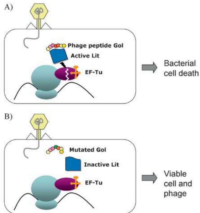
Figure 22: Le système Abi. A : Fonctionnement classique du système Abi qui entraîne la mort de la cellule infectée. B : Une mutation au niveau du polypeptide Gol réduit l'activation de la protéine Lit qui clive le facteur EF-Tu qui entraîne normalement la mort de la cellule. La cellule est maintenue viable, le virus peut réaliser une infection efficace (Stern et Sorek 2011).
