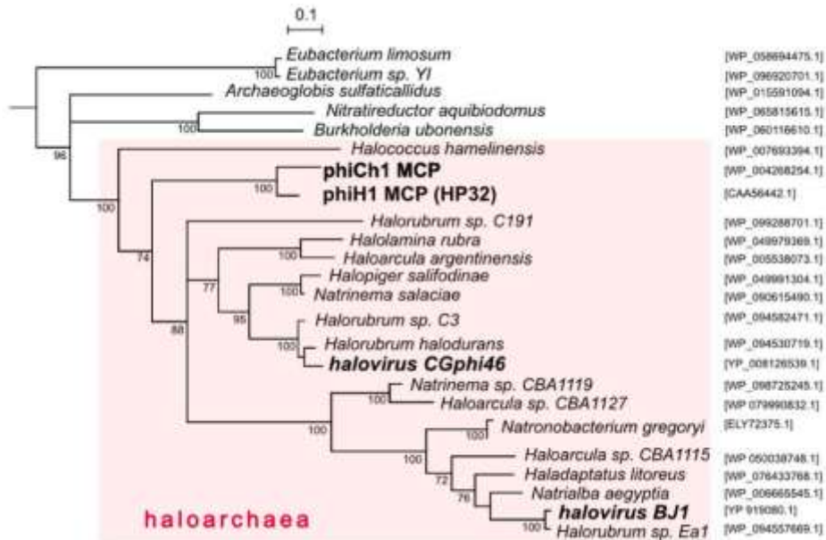
Figure 56 : Arbre phylogénétique obtenu à partir de la comparaison de la MCP (« Major Capsid Protein ») de ΦH, de virus halophiles et de protéines proches d'haloarchées (Dyall-Smith et al 2018).
