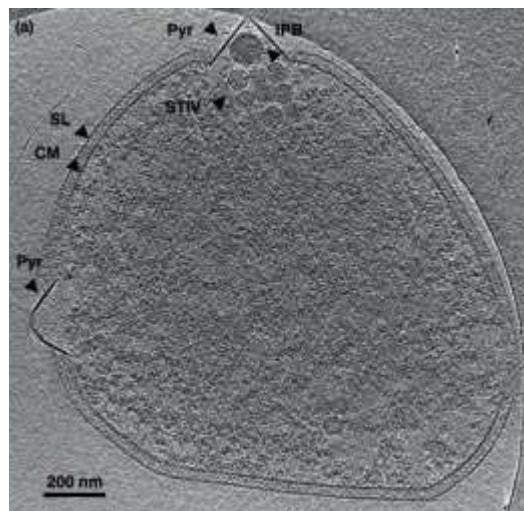
Figure 54 : Cryo-électromicroscopie d'une cellule de Sulfolobus infectée par STIV. Pyr = Structures Pyramidales ; PS = Espace périplasmique ; CM = Membrane cellulaire ; SL = S-Layer. (Fu and Johnson 2012).
