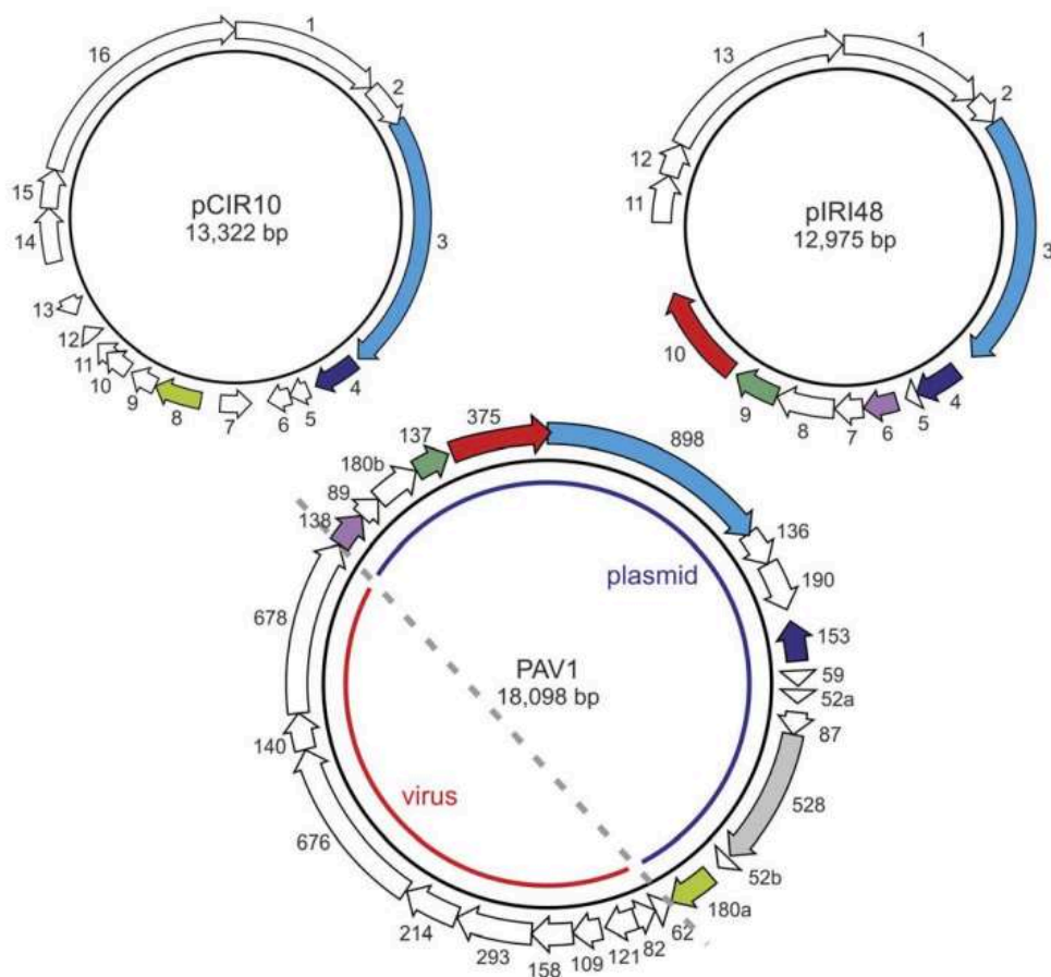
Figure 66 : Organisation génétique du génome de PAV1 et des plasmides de Thermococcales pCIR10 et pIRI48. Les gènes homologues sont représentés dans la même couleur (Krupovic et al 2013).
