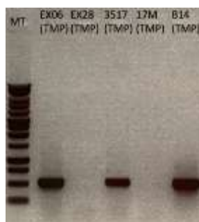
Figure 5 : Exemples de résultats PCR pour la TMP pour les souches EX 06, EX 28 140, 3517R1, 17Meth20 et B14-1.2.
