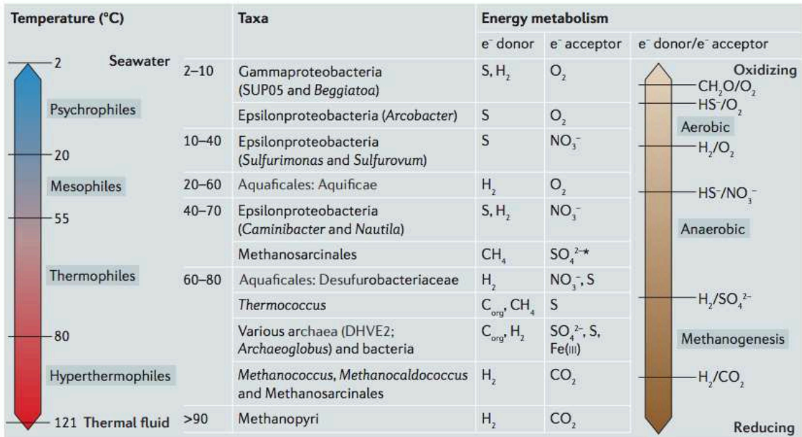
Figure 41 : Diversité microbienne retrouvée au niveau des sources hydrothermales océaniques profondes (Dick 2019).
