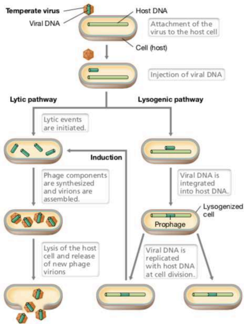
Figure 8: Cycles lytique et lysogénique (Madigan et al 2010).
