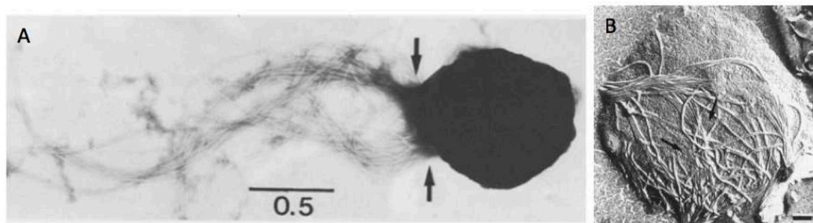
Figure 1 : A : Methanocaldococcus jannaschii JAL-1 en MET. Les flèches indiquent les deux lots de multiples flagelles situés à un pôle de la cellule. L'échelle représente 0,5 µm (Jones et al 1983). B : Methanocaldococcus vulcanius M7 T en MET. Les flèches indiquent les flagelles de la cellule. L'échelle représente 100 nm (Jeanthon et al 1999b).
