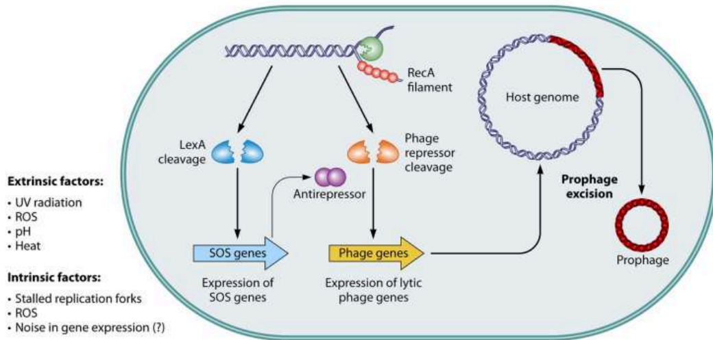
Figure 12: Un exemple d'induction spontanée dépendant du système SOS de l'hôte. Des facteurs intrinsèques et extrinsèques jouent un rôle sur l'état de l'ADN en induisant des dommages ou des blocages des polymérase laissant apparaître de l'ADN simple brin lié à des protéines RecA. Ce filament de nucléoprotéine déclenche le clivage de LexA ce qui conduit à l'expression des gènes SOS. Ainsi, la croissance cellulaire est inhibée et la réparation de l'ADN débute. Une autre voie consiste en l'inactivation de répresseurs des gènes viraux qui permet l'expression de gènes lytiques qui engendrent l'excision du prophage du génome de l'hôte, son empaquetage et sa libération de la cellule par lyse de celle-ci sous forme de virion (Nanda et al 2015).
