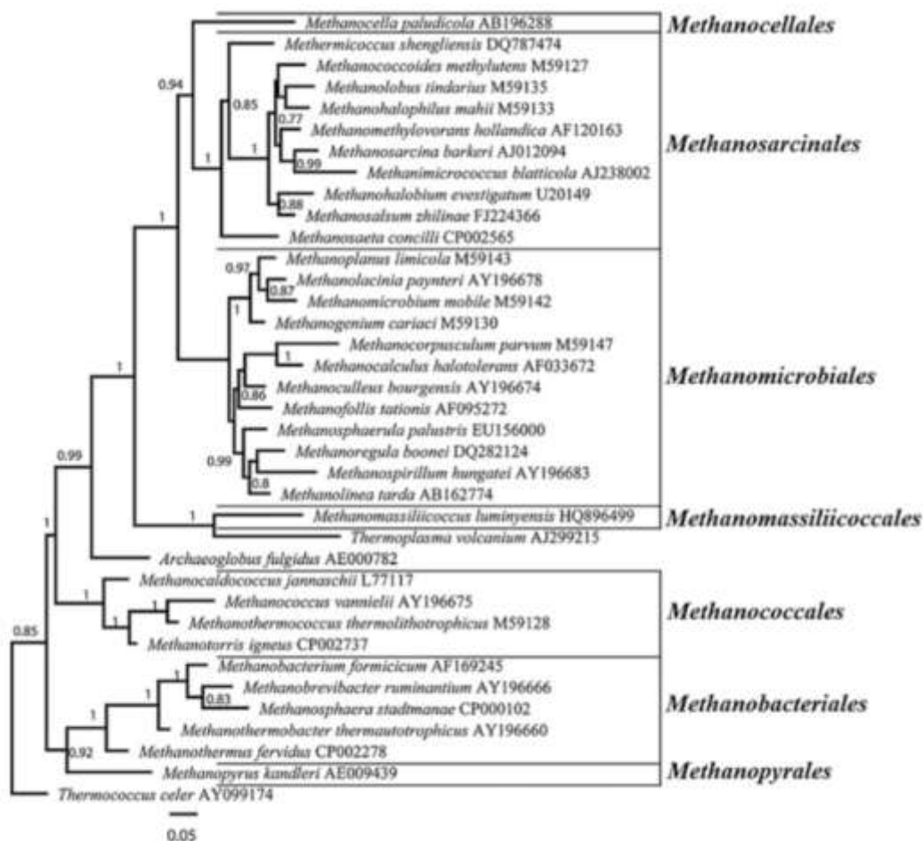
Figure 44 : Arbre phylogénétique basé sur la comparaison de séquences presque complètes de l'ARNr 16S, d'espèces types de 34 genres de méthanogènes (Lyu and Liu 2018).
