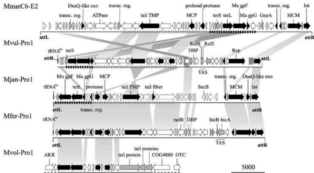
Figure 77 : Représentation comparative de l'organisation de différents génomes proviraux de Methanococcales (D'après (Krupovic et al 2010)).
