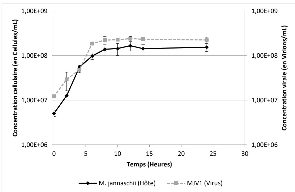
Figure 17 : Cinétique de croissance hôte-virus en conditions optimales de culture de M. jannaschii JAL-1 analysée en cytométrie en flux.
