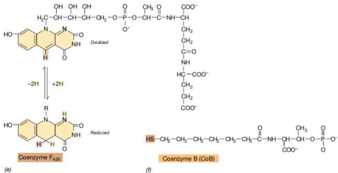
Figure 47 : Les coenzymes F420 et CoB ont la fonction de donneurs d'électron dans la réaction de méthanogénèse (Madigan et al 2010).
