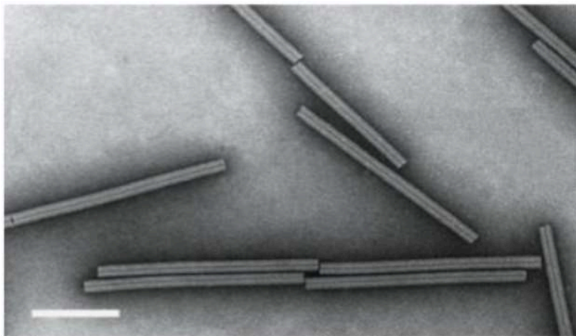
Figure 2: Photographie en microscopie électronique en transmission du virus de la mosaïque du tabac, barre d'échelle = 100 nm (Source ICTV).
