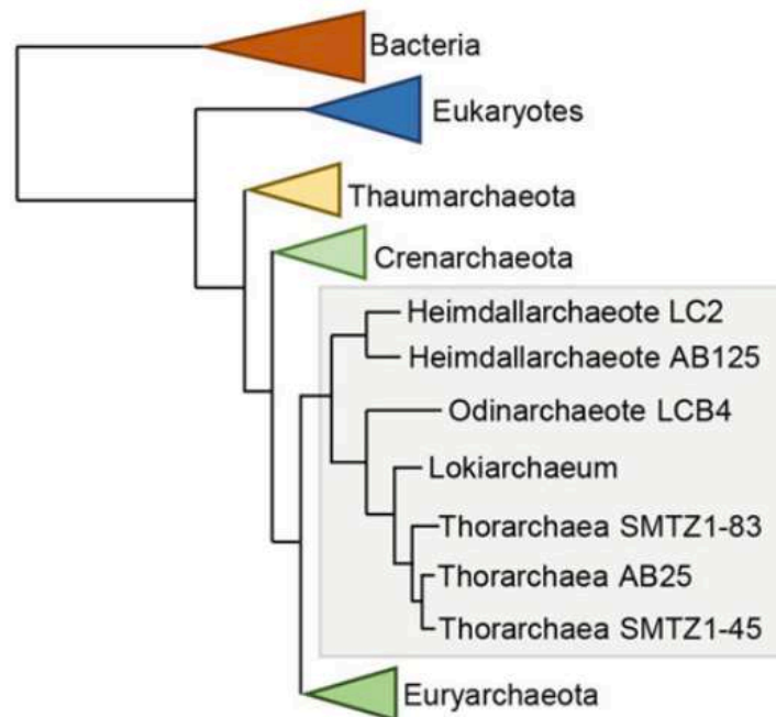
Figure 34 : Représentation schématique de la phylogénie obtenue suite à l'analyse de Da Cunha et ses collaborateurs (Gaia et al 2018).
