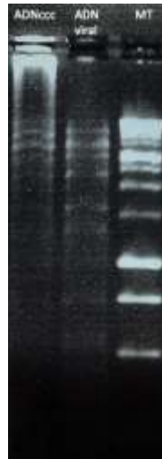
Figure 8 : Comparaison des profils de restriction obtenus à partir de l'ADNccc isolé de T. thioeducens UBOCC-M-2423 et de l'ADN viral obtenu à partir d'une fraction purifiée de virions issus de culture de T. thioeducens UBOCC-M-2423. MT : Le marqueur de taille = 1 kb DNA ladder, Promega.
