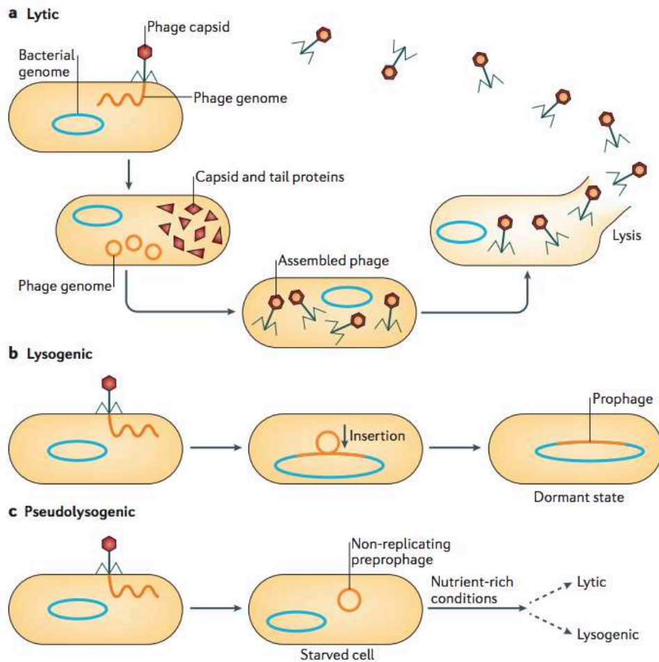
Figure 9: Description des cycles viraux classiques incluant la pseudolysogénie (Feiner et al 2015).
