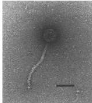
Figure 68 : \Psi M1 observé en microscopie électronique en transmission. L'échelle représente 70 nm (Jordan et al 1989).
