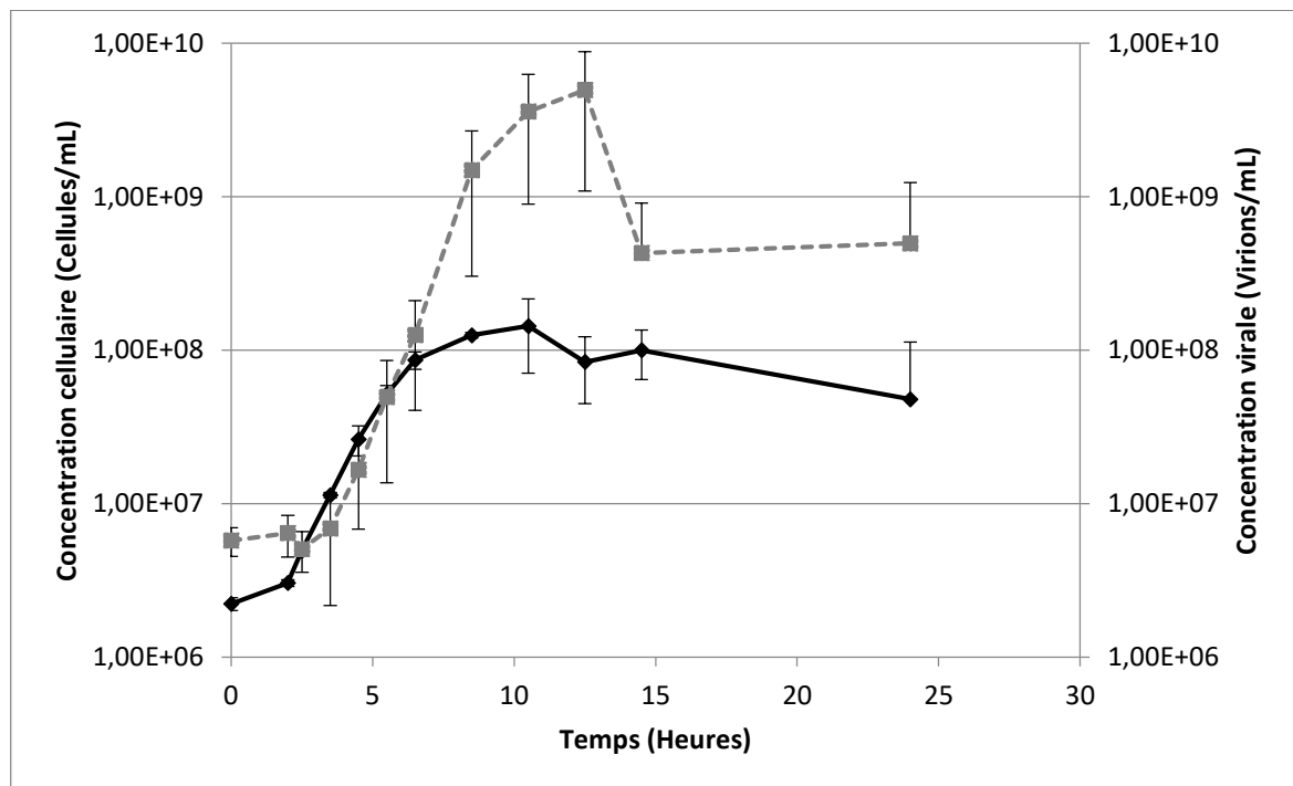
Figure 3 : Cinétique de croissance hôte-virus en conditions optimales de culture de T. thioeducens UBOCC-M-2423 analysée en cytométrie en flux. En noir : croissance cellulaire de T. thioeducens UBOCC-M-2423. En gris : Production virale basale du Thiovirus.
