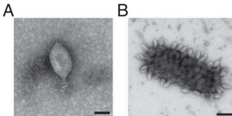
Figure 1: Les virions de NSV1 observés en MET. A. Le morphotype citron de NSV1. B : Les virions attachés à une cellule de Nitrosopumilus souche SW. La barre d'échelle représente 50 nm. (Kim et al 2019)
