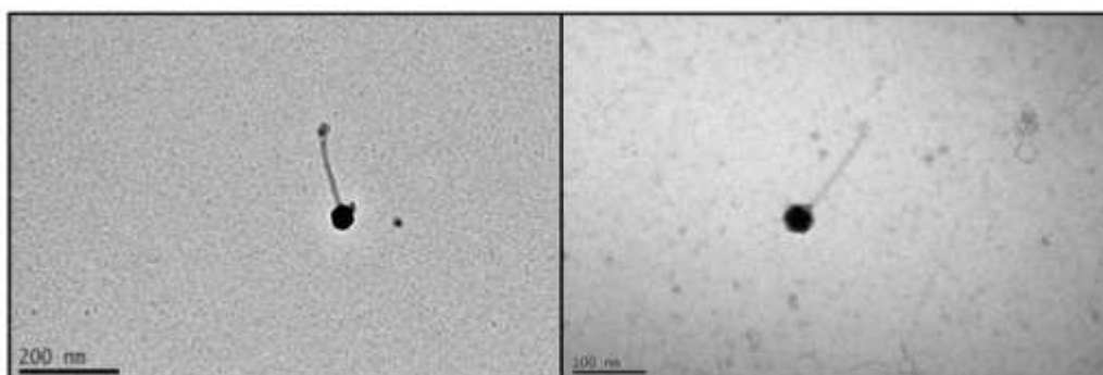
Figure 22 : Observation en MET d'une fraction purifiée de particules de types virales obtenues à partir de M. vulcanius M7 T .
