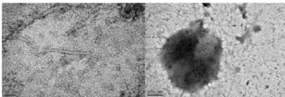
Figure 7 : Observation en MET d'une fraction concentrée obtenue à partir de cultures de la souche 3517R1.
