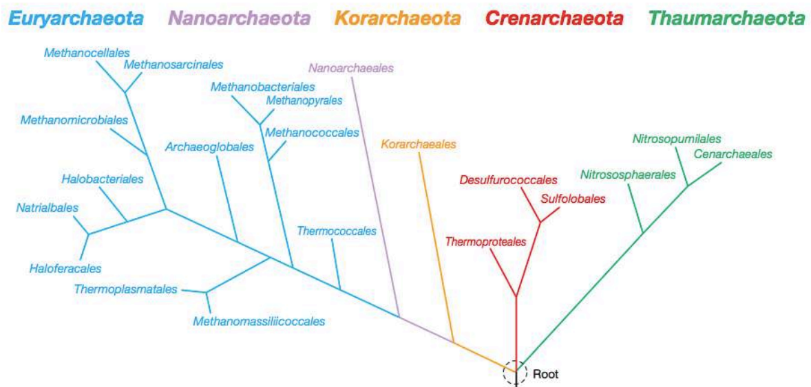
Figure 31 : Phylogénie des archées (Madigan et al 2010).
