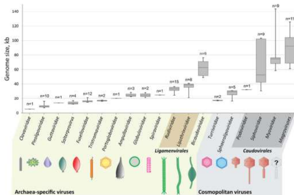
Figure 49 : Diversité morphologique des virus d'archées et distribution de la taille des génomes correspondant à chaque groupe de virus (Krupovic et al 2018).
