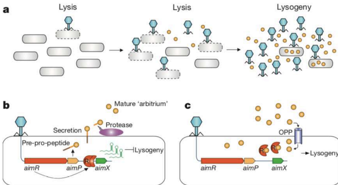
Figure 10: Modèle de décision de lyse-lysogénie basé sur la communication entre virus. a : Dynamique de l'accumulation d'arbitrium lors de l'infection d'une culture bactérienne par un phage. b : Première rencontre du phage avec une population bactérienne, les gènes aimR et aimP sont exprimés suite à l'infection. AimR, en tant que dimère, active l'expression de AimX qui est un inhibiteur de la lysogénie (éventuellement sous la forme d'un ARN régulateur non-codant) dirigeant le phage vers un cycle lytique. AimP est également exprimé, sécrété et traité de manière extracellulaire pour produire le peptide mature « arbitrium ». c : Plus tard durant l'infection, le peptide arbitrium s'accumule dans le milieu et est internalisé dans la bactérie par le transporteur OPP. Lorsque le phage infecte la bactérie, le récepteur AimR exprimé se lie aux molécules d'arbitrium et ne peut pas activer l'expression de AimX, ce qui permet l'entrée en cycle lysogénique (Erez et al 2017).
