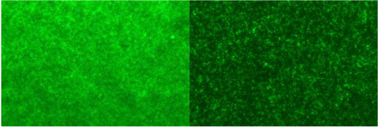
Figure 23 : Observation d'une solution concentrée de VLPs obtenu à partir de cultures de M. fervens AG86 en microscopie à épifluorescence. A gauche : Dilution 1000, à droite : dilution 10 000.
