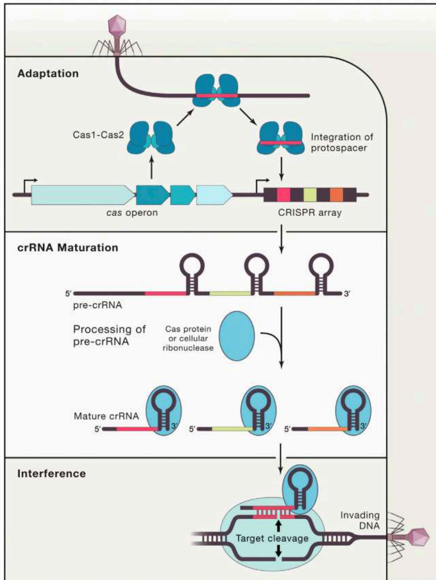
Figure 20: Les trois phases du système d'immunité CRISPR (Hille et al 2018).
