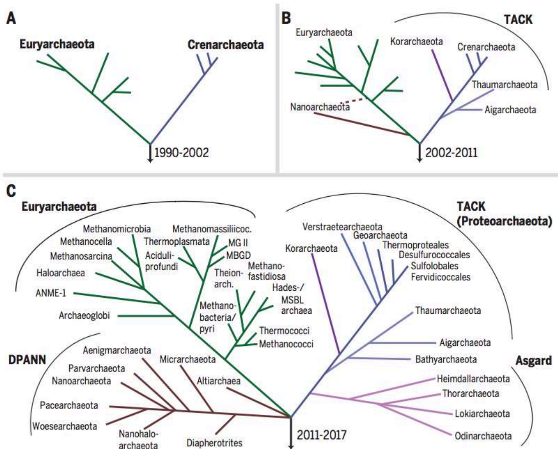
Figure 32 : Evolution de la classification des archées au cours des trente dernières années (Spang et al 2017).
