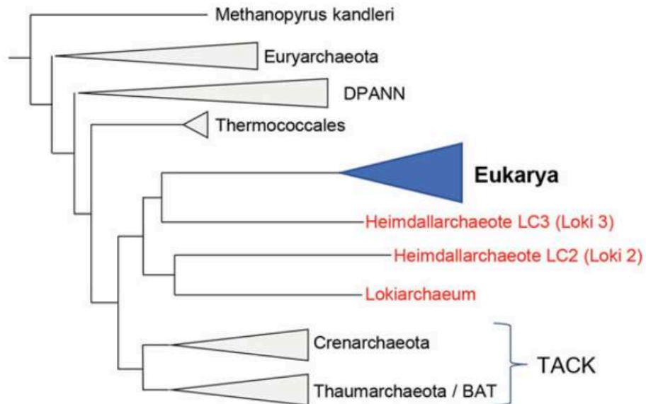
Figure 33 : Représentation schématique de la phylogénie obtenue suite à l'analyse de Spang et ses collaborateurs (Gaia et al 2018).
