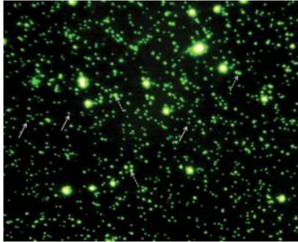
Figure 24: Photographie de microscopie à épifluorescence d'échantillon d'eau de mer marqué au SYBR Green. Les virus sont indiqués par une flèche pleine et les bactéries par une flèche en pointillés (Suttle and Fuhrman 2010).
