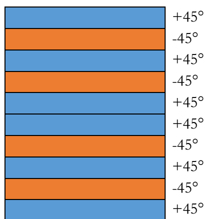
Fig. 2-3: C/PEKK ply stacking
