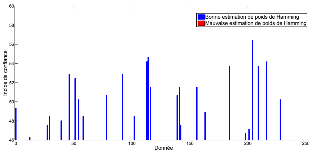
FIGURE 2.13 – Résultat de l'amélioration de l'algorithme du K-means pour les plus hauts indices de confiance
