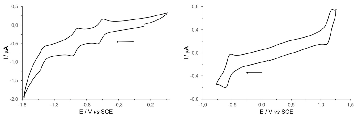
Figure 6. Voltammogrammes cycliques mesurés pour le fulléropillar[5]arène 1 dans \text{CH}_2\text{Cl}_2 + 0,1 M n\text{-Bu}_4\text{NBF}_4 à une vitesse de balayage de 200 mV/s.
