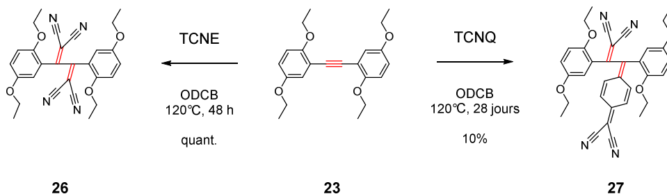
Schéma 28. Réactions de cycloadditions [2+2] par voie thermique sur le modèle 23 avec le TCNE et TCNQ.
