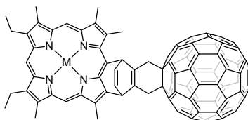
Schéma 1. Première synthèse d'une dyade C 60 -porphyrine par le groupe de Devens Gust et col. en 1994.
