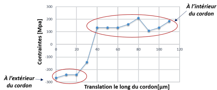
FIGURE 5.8: Contraintes résiduelles le long d'un cordon de soudure verre/silicium soudé par impulsions laser nanosecondes ( \lambda = 1027 \text{ nm} , f = 29 \text{ kHz} , P_{\text{moy}} = 11,25 \text{ W} , v = 24 \text{ mm/s} )
