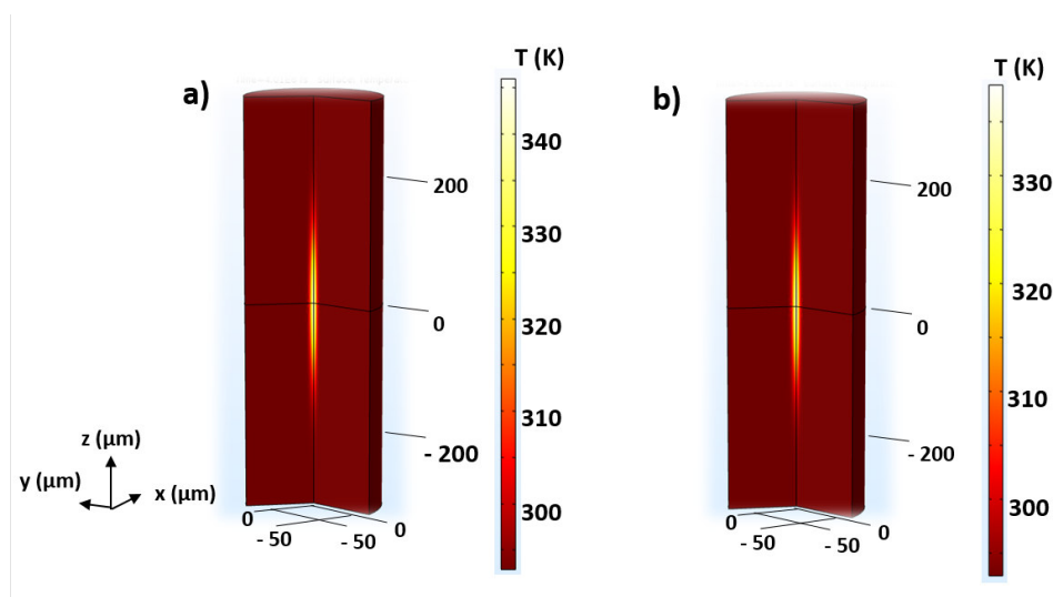
FIGURE 5.3: Élévation de température dans le verre due à l'absorption d'une impulsion sur un diamètre de 15 \mu\text{m} et une profondeur de 300 \mu\text{m} . a) Température maximale atteinte lors de l'absorption de l'impulsion. b) Température après diffusion de la chaleur dans le verre durant 2 \mu\text{s} .
