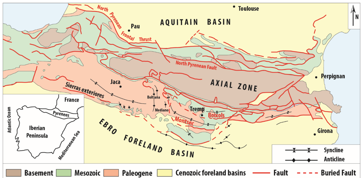
Fig.2.1: carte géologique simplifiée des Pyrénées mettant en évidence les différents domaines, les grands accidents tectoniques (modified from Munoz, 1992)
