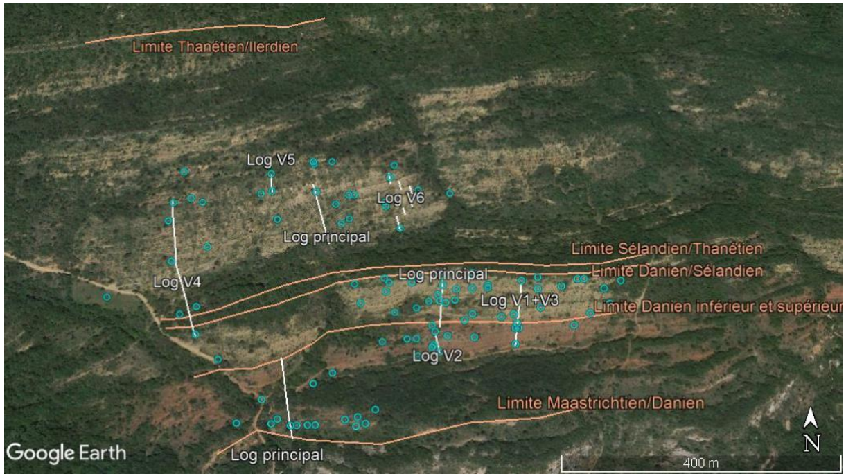
Fig. 4.21 : localisation des coupes réalisées et de tous les points GPS pris dans le Paléocène de la région de Lairyère
