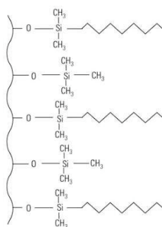
Figure 23 : Phase stationnaire Zorbax Eclipse plus avec double post-silanisation (source : www.agilent.com ).
