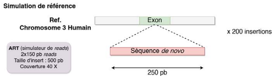
FIGURE 4.1 – Simulation de référence. 200 insertions de novo sont générées dans le chromosome 3 du génome humain Hg38.
