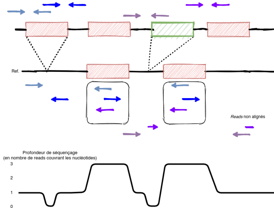
FIGURE 2.4 – Informations d’alignement produites par les variants de structure. Les signaux produits par les insertions sont plus contrastés que ceux des délétions. Les insertions de type duplicative (en rouge) induisent une distance entre paire de reads plus grande qu’attendue. Les reads associés à une duplication ont un risque d’être alignés de multiple fois sur le génome ( reads encadrés). Ces informations ne sont pas observables avec des insertions de novo (en vert) car une des paires ou une partie d’un read ne s’aligne pas sur le génome de référence. L’ensemble des insertions produisent une perte de profondeur de séquençage locale au niveau des points de cassure. Les insertions de type duplicative induisent une augmentation de la profondeur de séquençage au niveau des copies de l’insertion.
