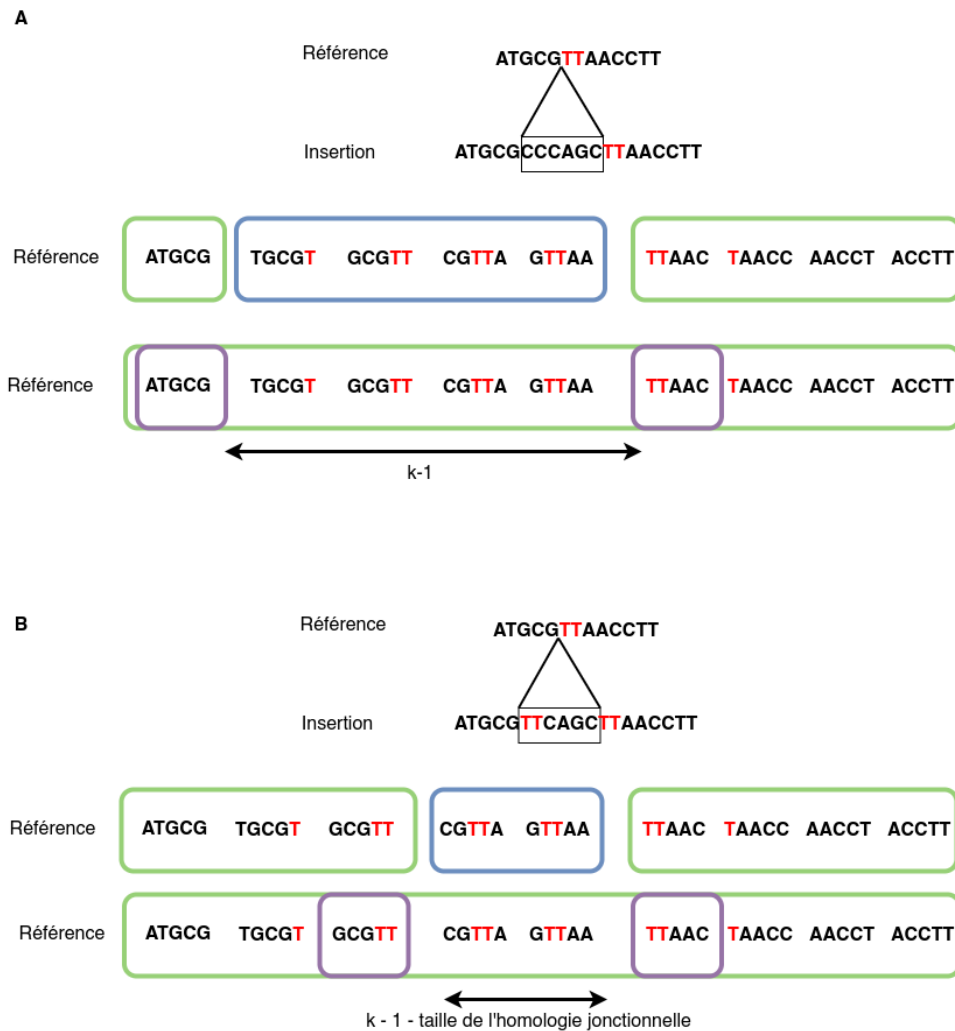
FIGURE 5.3 – Impact des homologies jonctionnelles sur les signature des insertions homozygotes et hétérozygotes dans MindTheGap. Schéma comparant l’impact d’une homologie jonctionnelle de taille 2 (TT, en rouge) sur les motifs des insertions homozygotes et hétérozygotes. Les k-mers du génome de référence absents dans le graphe de De Bruijn sont encadrés en bleu, ceux présents en vert et ceux qui sont branchants en violet. A : motifs attendus pour des insertions homozygotes et hétérozygotes sans homologies jonctionnelles. B : altération des motifs décrit en A par la présence d’une homologie jonctionnelle de taille 2.
