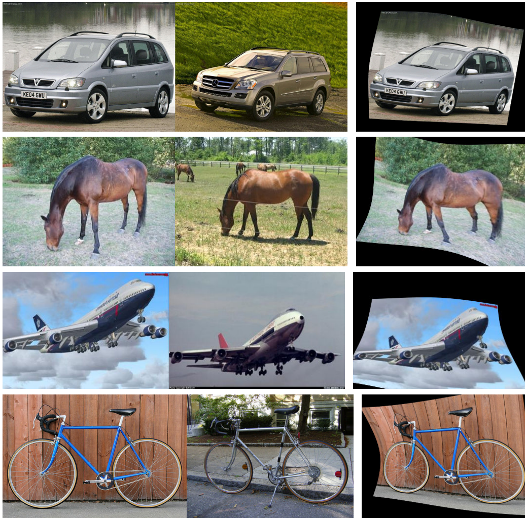
(b) TSS
