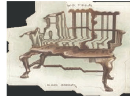
Output
