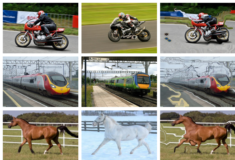
(b) TSS
