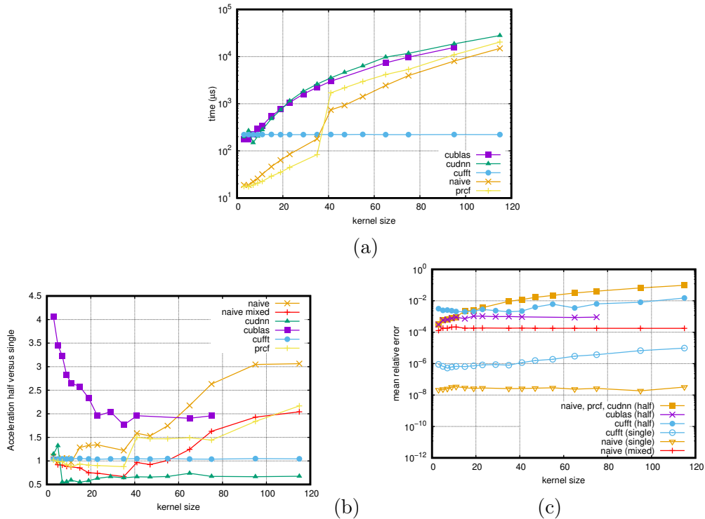
FIGURE 3.2 – Convolution 2D effectuée sur GPU volta-Titan sur des images de taille 512 \times 512 avec différentes tailles de noyau en abscisse : (a) temps de calcul en flottant simple précision ; (b) accélération avec les calculs effectués en demi-précision par rapport aux calculs effectués en simple précision ; (c) erreur de calcul par rapport à une implémentation sur CPU en double précision.
