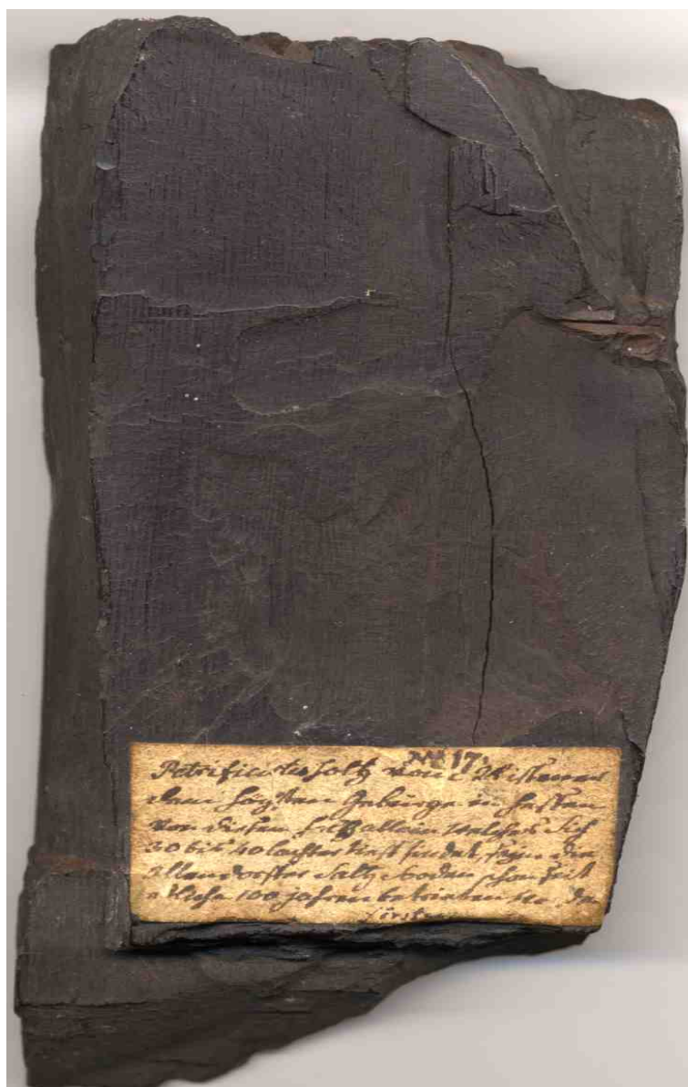
Figure 58. Les pratiques d'étiquetage au sein de la collection minéralogique de Jean Hermann 1398
