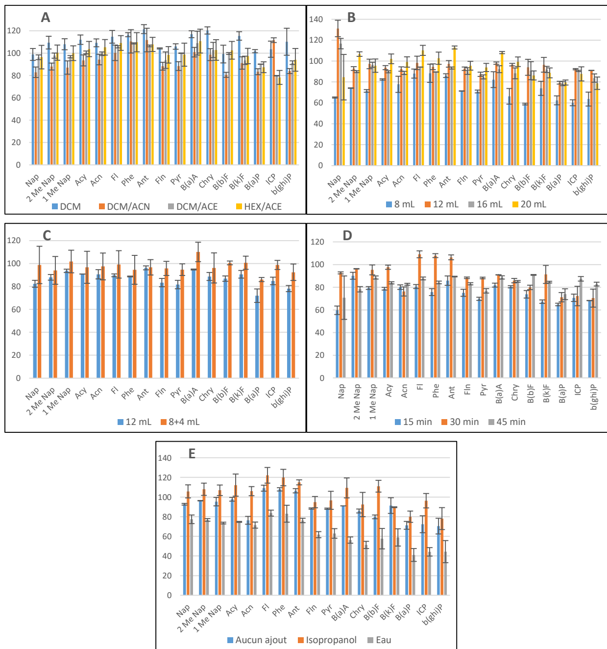
Figure 2.5: les rendements d'extraction de 17 HAPs à partir de sol dopé à 150 ng.g -1 pour les différents paramètres optimisés: (A) le solvant d'extraction, (B) le volume de solvant, (C) le fractionnement du solvant, (D) la durée d'extraction et (E) l'effet de l'eau et l'isopropanol.
