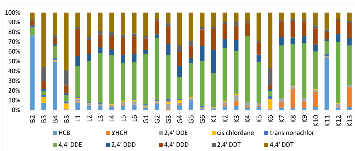
Figure 5.7: La contribution en pourcentage des OCPs les plus fréquemment détectés.
