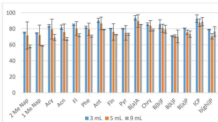
Figure 2.8: Choix du volume de DCM utilisé pour l'éluion des HAPs.
