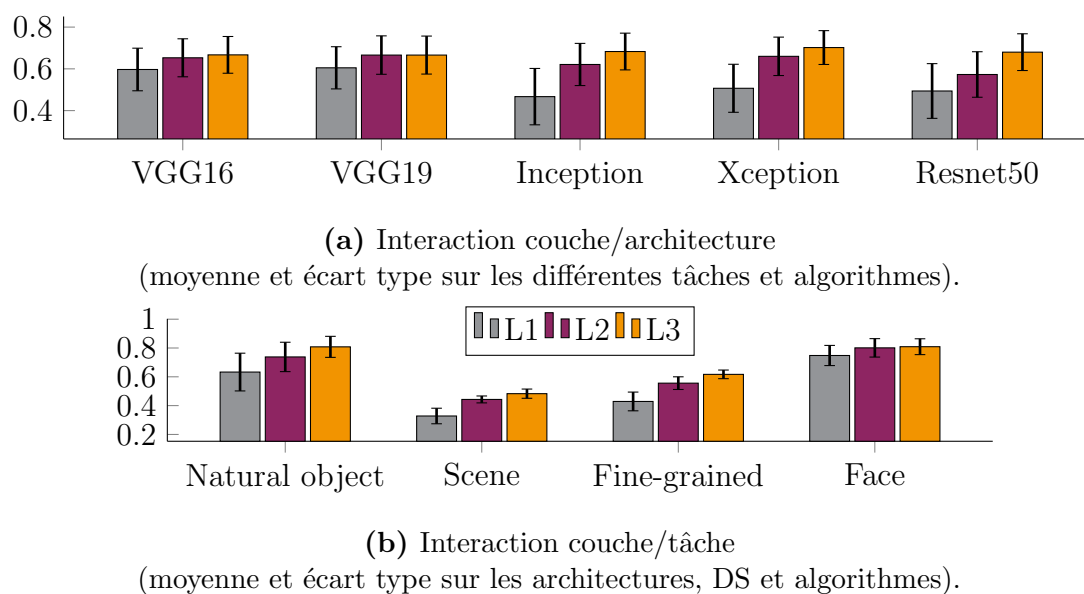
Figure G.8: Influence de la couche d'extraction sur le partitionnement (NMI).
