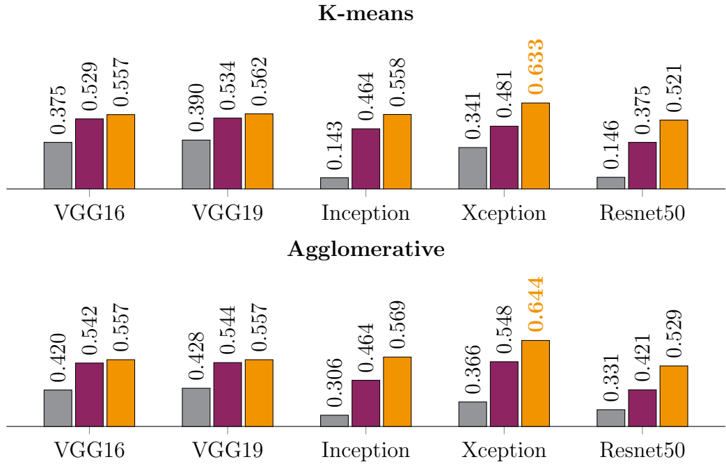
(b) Birds
