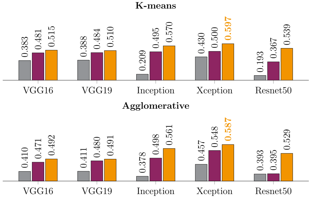
(b) MIT
