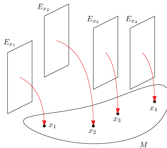
Figure 1.3: Un fibr  vectoriel de rang 2 de base M :   chaque point x \in M est associ  une copie E_x du plan \mathbb{R}^2 .
