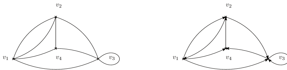
Figure 1.11: À gauche : un graphe admissible non orienté plongé dans le plan. À droite : une orientation possible de ce même graphe.
