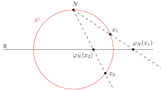
Figure 1.2: La projection stéréographique par rapport au pôle Nord dans la sphère S^1 \subset \mathbb{R}^2 .
