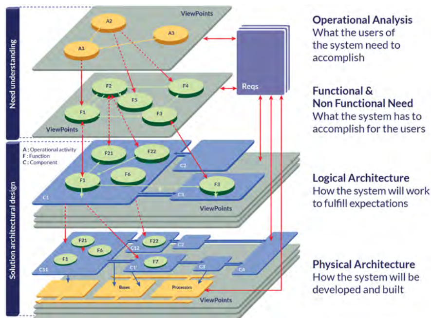
FIGURE 2.16 – Les 4 principales couches systèmes de la méthode ARCADIA [Cla19].
