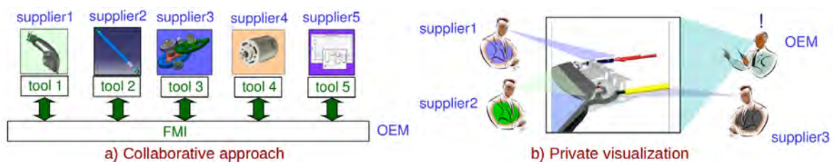
FIGURE 2.22 – Les aspects « collaboratif » et « privé » du standard FMI 2.0 [FMI14].
