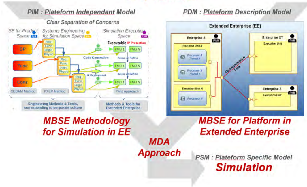
FIGURE 1.1 – Vue d’ensemble des propositions, avec l’approche MDA.
