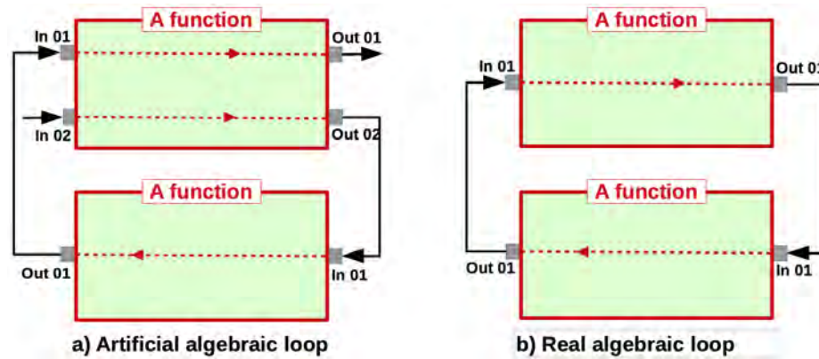
FIGURE 3.23 – Différentes boucles algébriques [FMI14]
