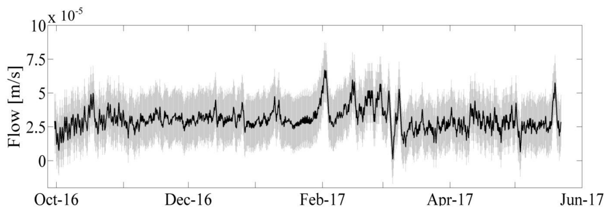
Figure 3-19. Estimation des flux à partir des données de température collectées avec le profil PVT 1. La courbe noire présente l'estimation pour \lambda=2.5 \text{ W/m/K} et la zone grise représente la gamme de flux estimés pour des valeurs de \lambda allant de 1 à 4 \text{W/m/K} (les valeurs de flux estimées les plus fortes étant associées à \lambda=4 \text{ W/m/K} ). Une valeur positive de flux implique un flux vertical descendant.
