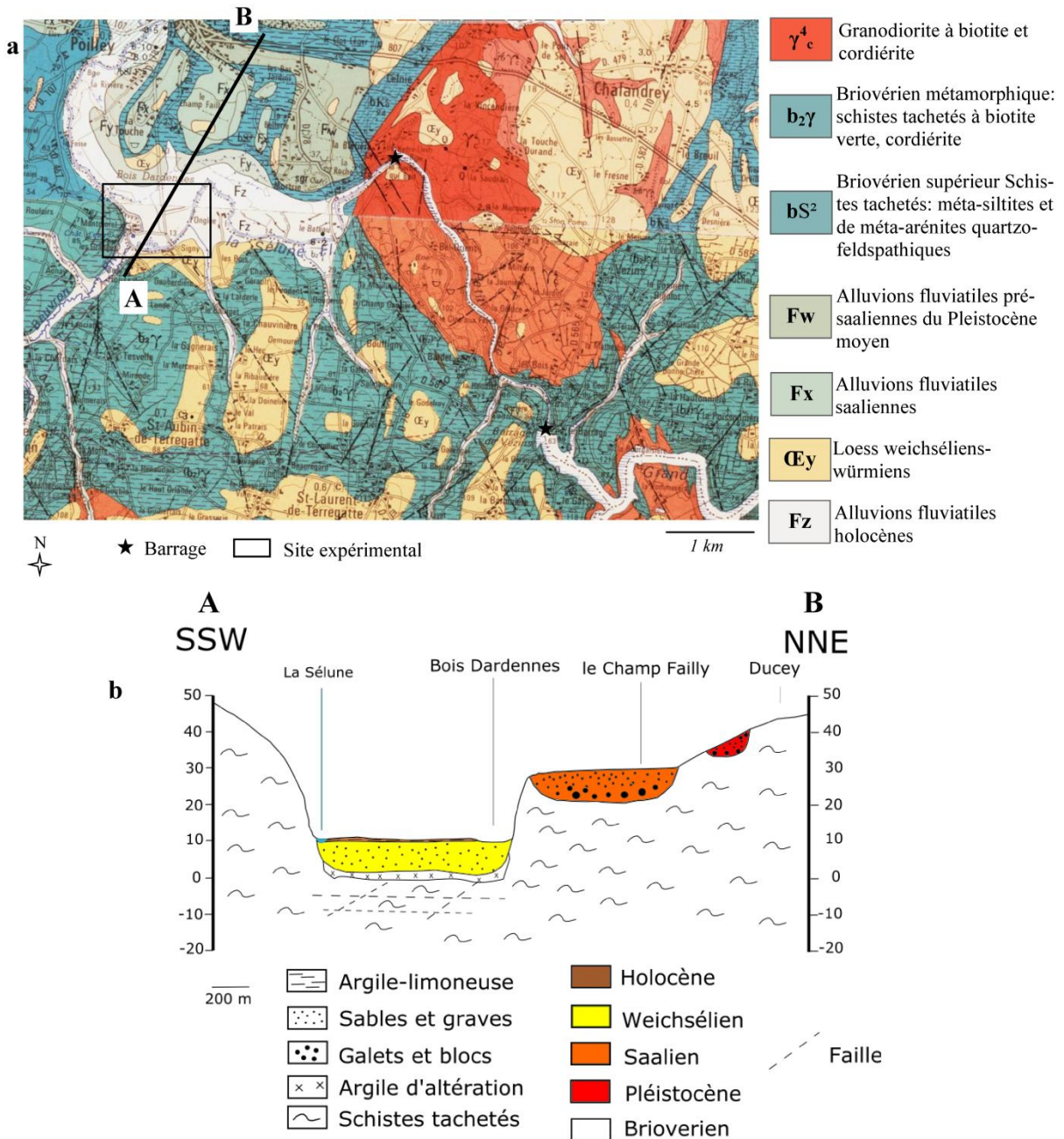
Figure 3-8. a. Carte géologique à l'échelle 1/50 000 du site expérimental (rectangle noir) et de sa région proche [modifiée depuis Beurrier et al. (1984) et Dadet et al. (1983)]; b. Coupe géologique de la plaine alluviale depuis le pont de Signy jusqu'à la commune de Ducey [modifiée depuis Robustelli et al., (2018)]
