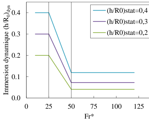
Figure 55 : Modèle de l'évolution de la hauteur d'immersion dynamique avec Fr^* .
