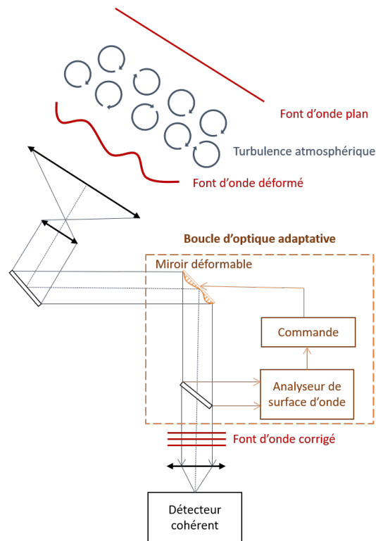
FIGURE 2.4 – Principe de fonctionnement d'une boucle d'optique adaptative
