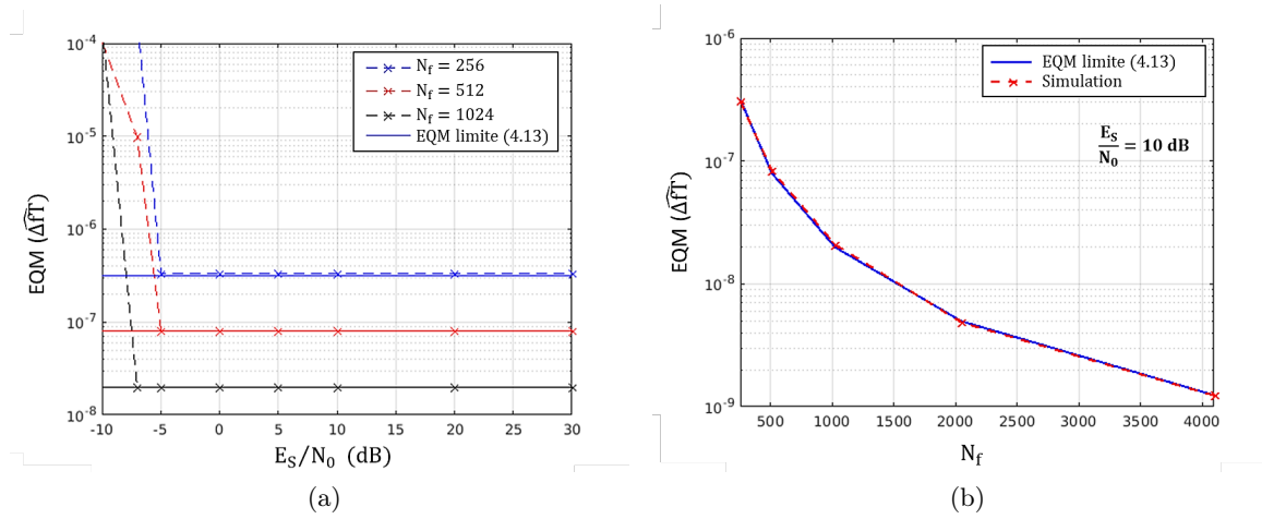
FIGURE 4.2 – (a) EQM \mathbb{E}[|\Delta f T - \widehat{\Delta f T}|^2] de l'écart en fréquence résiduel en fonction de E_S/N_0 pour différentes tailles de blocs N_f . (b) EQM en fonction de N_f pour E_S/N_0 = 10 dB. Les courbes simulées sont comparées à la limite théorique (4.13) ( \Delta f = 100 MHz, T=0.1 ns).
