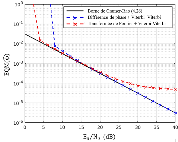
FIGURE 4.17 – Évolution de l'EQM de la phase résiduelle en fonction du RSB pour les deux systèmes de synchronisation en boucle ouverte (Modulation BPSK, N_f=512 , N_p=16 , \Delta f=100 MHz) sans bruit de phase laser. La figure illustre l'apparition d'un plancher d'erreur à fort RSB pour la méthode basée sur la transformée de Fourier discrète.
