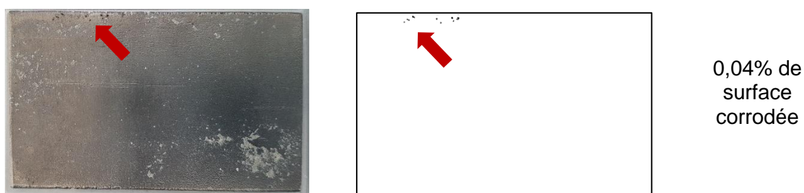
Figure 59 - Apparition de produits de corrosion à 3 jours d'hydratation pour un mélange 50/50 activé à 0,4% Cl- (les pourcentages de surfaces corrodées apparentes sont déterminés par traitement d'image)
