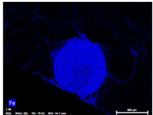
Cartographie EDS du Fer
