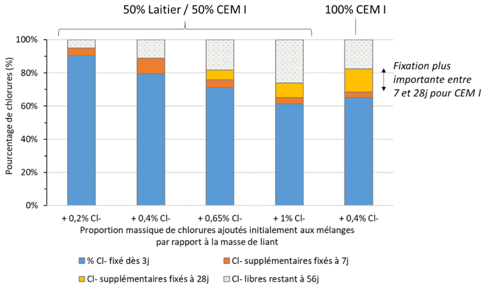
Figure 138 - Bilan de masse en chlorures libres par rapport à la quantité totale de chlorures ajoutée en fonction de l'activation
