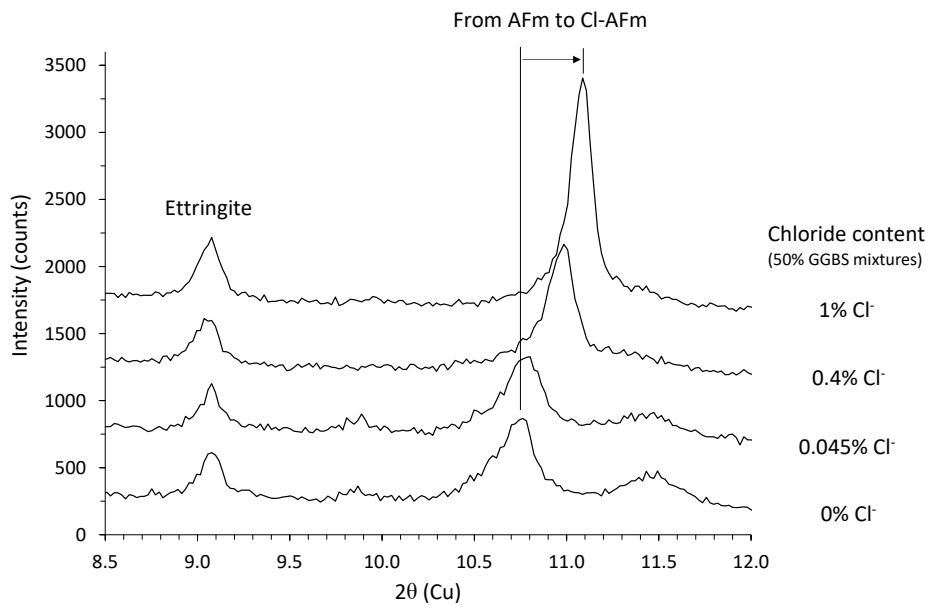
Figure 142 – Diagramme DRX à 120 jours d'hydratation de matrice à base de 50% de laitier et 50% de CEM I actives avec une teneur croissante en chlorures (NaCl)
