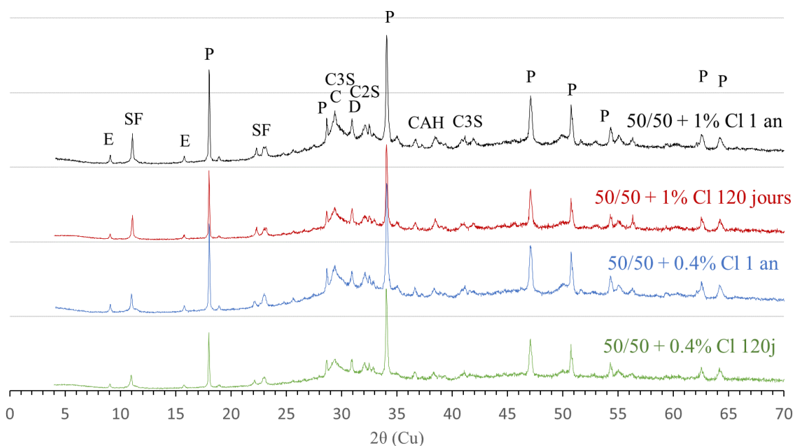
Figure 145 – Diffractogrammes à 120 jours et 1 an d'hydratation sur pâtes contenant 50% de laitier de haut-fourneau et deux teneurs en chlorures 0,4 et 1% (E: ettringite; SF : Sel de Friedel, P: portlandite, D : Dolomite, C : calcite)
