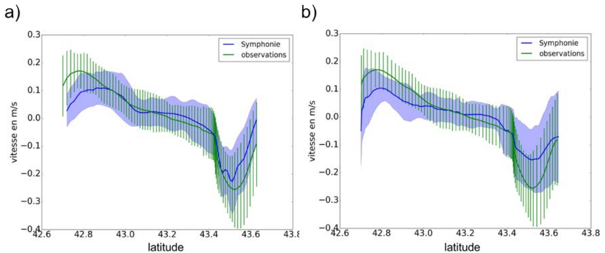
FIGURE 4.5 – Profil moyen des courants perpendiculaires à la trajectoire des gliders le long de la radiale Nice-Calvi pour Symphonie a) OLYMPE1 et b) S-WM111_23052015 (en bleu) et les gliders (en vert). L'écart-type est représenté par les barres d'erreur (pour les radars) et l'enveloppe (pour le modèle).
