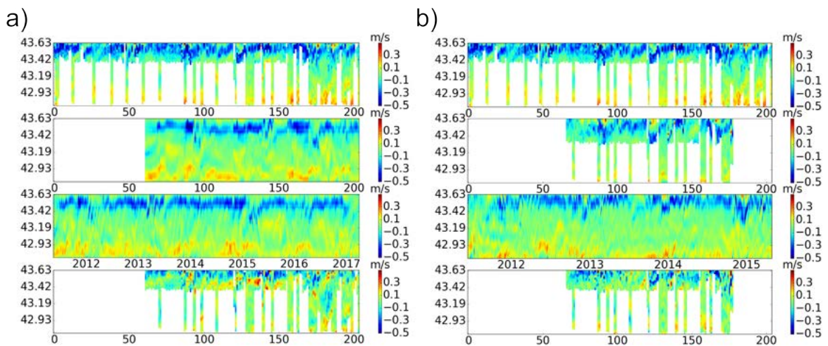
FIGURE 4.6 – Courants géostrophiques pour les gliders (1 er diagramme), pour Symphonie avec la méthode des gliders pour les dates gliders (2 ème diagramme), Symphonie avec la méthode des méthode gliders pour les dates Symphonie (3 ème diagramme), Différences entre les deux premiers diagrammes (4 ème diagramme) pour la simulation a) OLYMPE1 et b) S-WM111_23052015.
