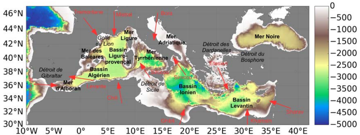
FIGURE 1.6 – Carte de la bathymétrie de la mer Méditerranée avec les noms des mers, détroits, bassins et vents
