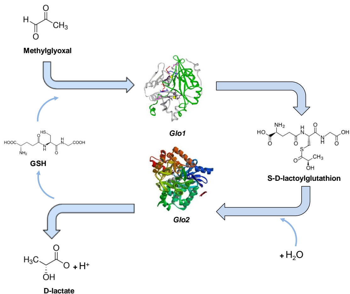
Figure 11 Le système glutathion/ glyoxalase, impliqué dans la métabolisation du méthylglyoxal.
