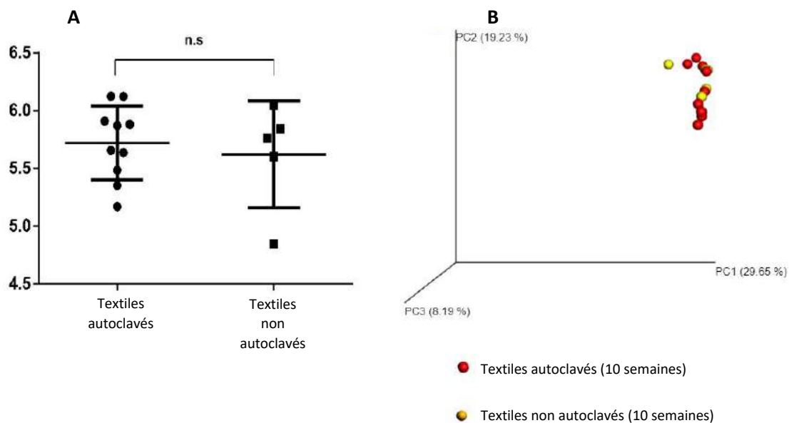
Figure 30 : Représentation de la diversité \alpha (A) et de la diversité \beta (B) des textiles exposés 10 semaines autoclavés ou non-autoclavés. L'ACP a été réalisée à partir de l'indice de Bray-Curtis.
