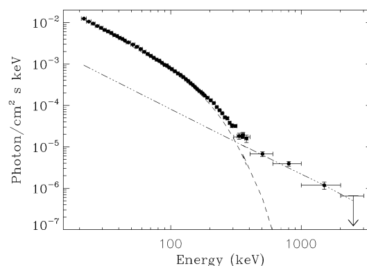
Figure 6.3 – Spectre dur de Cyg X-1 obtenu grâce au mode Compton (Laurent et al., 2011).
