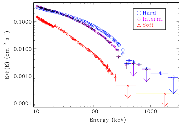
Figure 6.5 – Spectres des états dur, intermédiaire et mou de Cyg X-1 obtenus au mode Compton ( Rodriguez et al., 2015b ).
