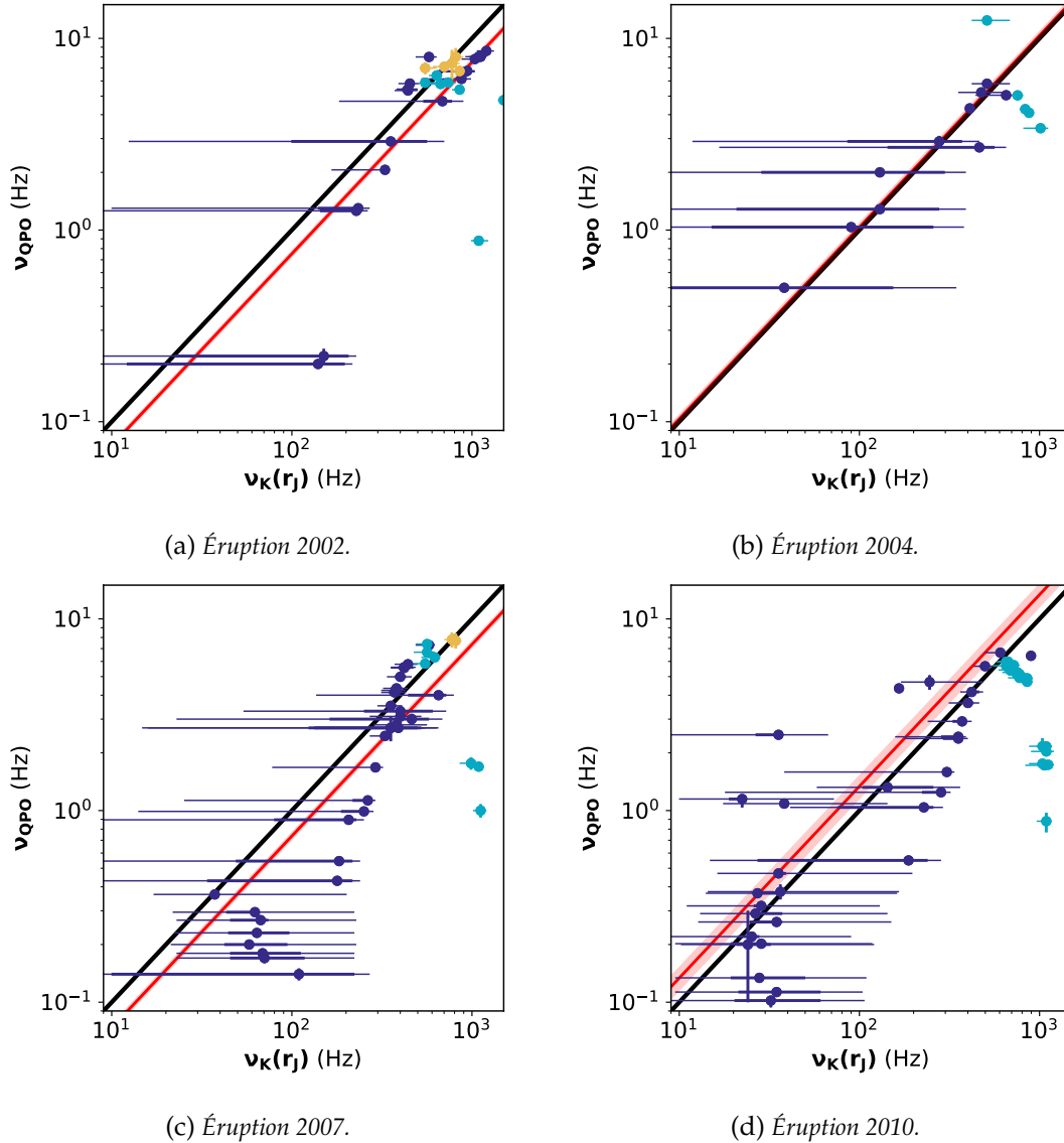
Figure 5.9 – Corrélation entre la fréquence des QPOs observés \nu_{\text{QPO}} et la fréquence képlerienne au rayon de transition \nu_K(r_J) pour chacune des éruptions.
