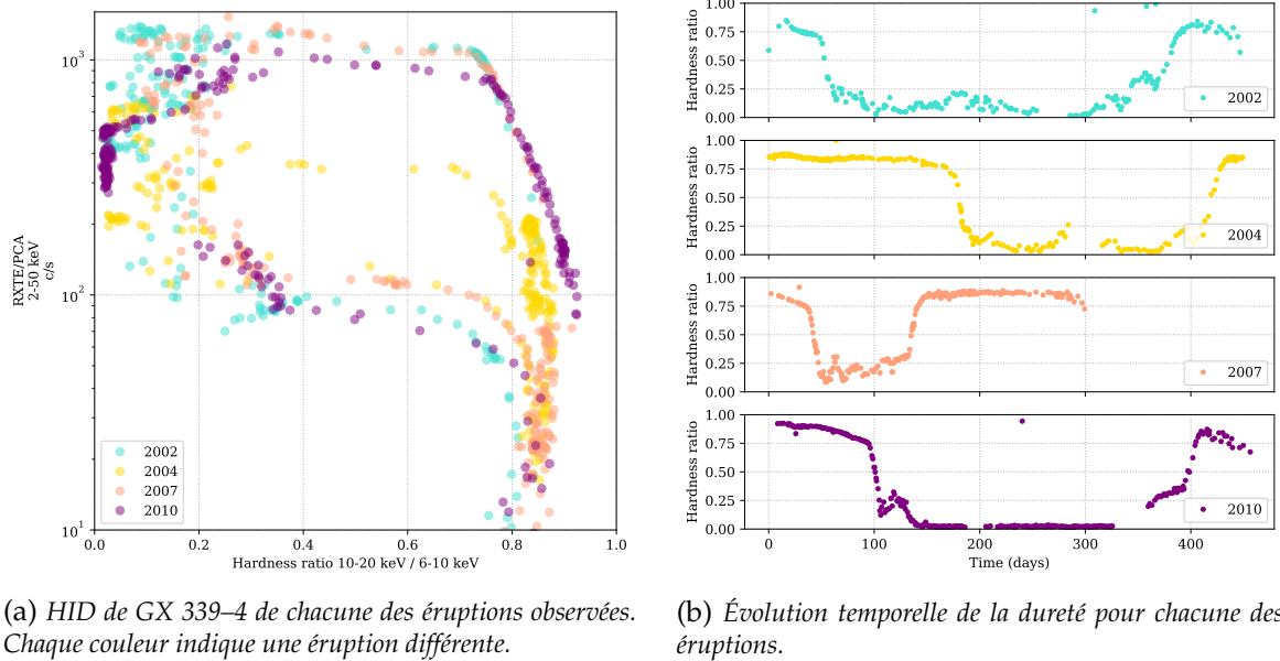
Figure 5.1 – Suivi de quatre éruptions de GX 339–4 obtenu à partir des données de RXTE/PCA.
