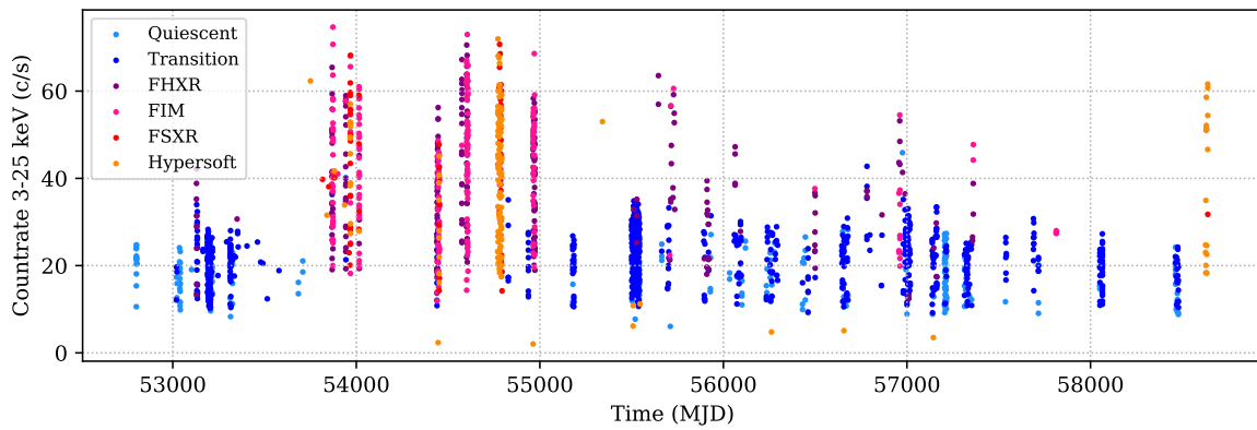
Figure 7.9 – Courbe de lumière JEM-X dans la bande 3–25 keV de Cyg X-3.
