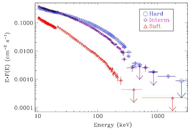
Figure 6.5 – Spectres des états dur, intermédiaire et mou de Cyg X-1 obtenus au mode Compton (Rodriguez et al., 2015b).
