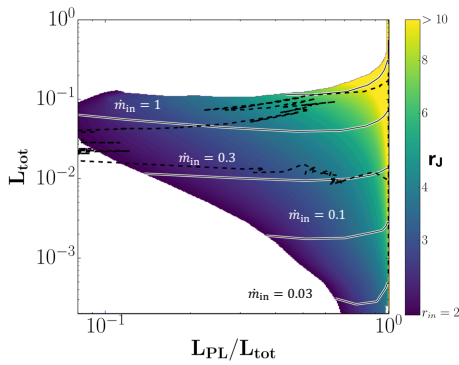
(a) L'échelle de couleurs indique l'évolution du rayon de transition r_j et les contours indiquent différentes valeurs du taux d'accrétion \dot{m}_{\text{in}} .
