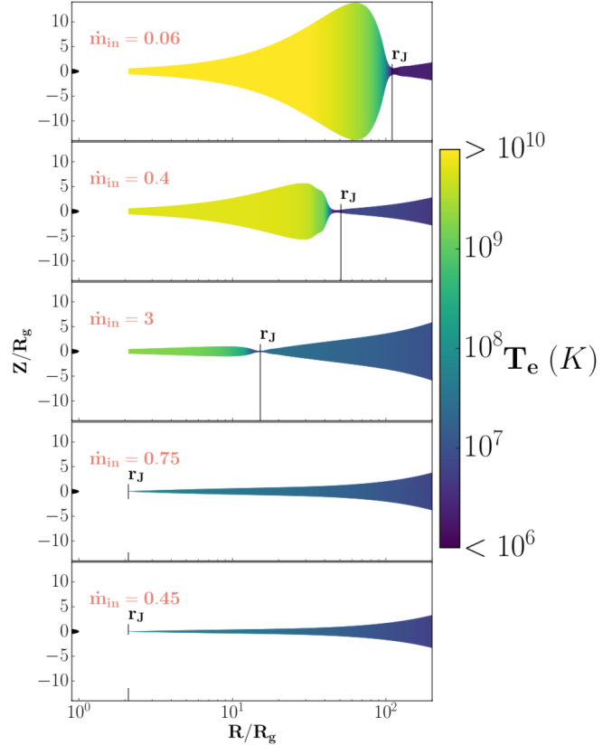
(c) Différentes configurations du disque hybride en fonction des paramètres r_j et \dot{m}_{\text{in}} . L'échelle de couleurs indique la température des électrons en Kelvin.
