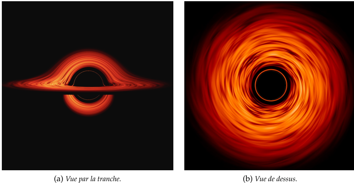
Figure 1.6 – Simulation de l'apparence d'un trou noir et de son disque d'accrétion distordu par effet de lentilles gravitationnelles. Credits : National Aeronautics and Space Administration (NASA) 's Goddard Space Flight Center/Jeremy Schnittman. La toute première simulation a été réalisée par Jean-Pierre Luminet en 1979 (Luminet, 1979).
