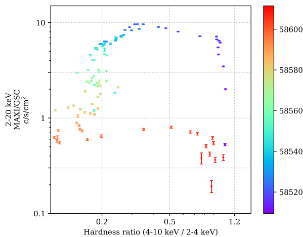
Figure 4.2 – HID de MAXI J1348–630. La carte de couleur retrace l'évolution temporelle en MJD.
