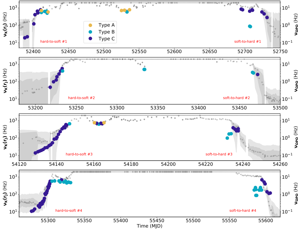
Figure 5.7 – Co-évolution de la fréquence observée des QPOs \nu_{\text{QPO}} et de la fréquence képlerienne \nu_K(r_j) pour les quatre éruptions étudiées.
