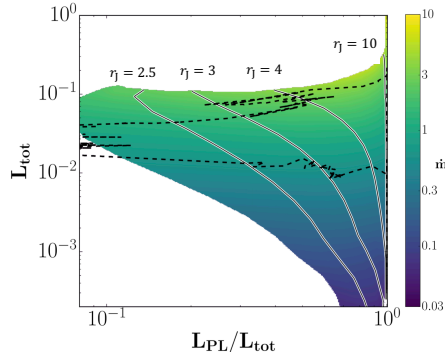
(b) L'échelle de couleurs indique l'évolution du taux d'accrétion et les contours indiquent différentes valeurs du rayon de transition r_j .
