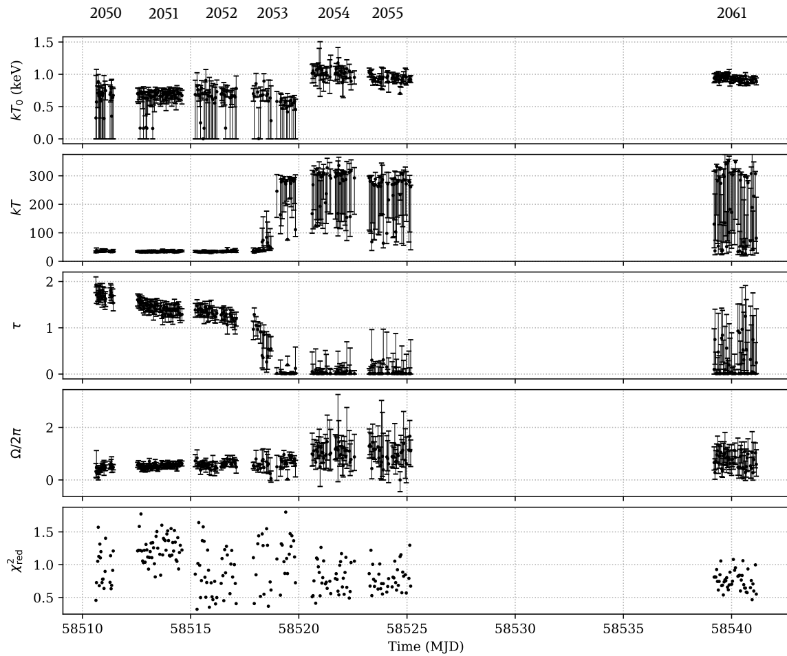
Figure 4.6 – Évolution des paramètres du modèle de Comptonisation au cours de l'éruption.
