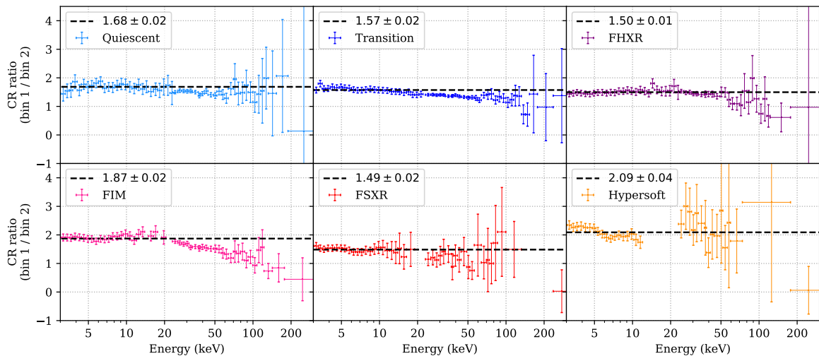
Figure 7.14 – Rapport des taux de comptage des spectres entre deux conjonctions pour chacun des états de Cyg X-3.
