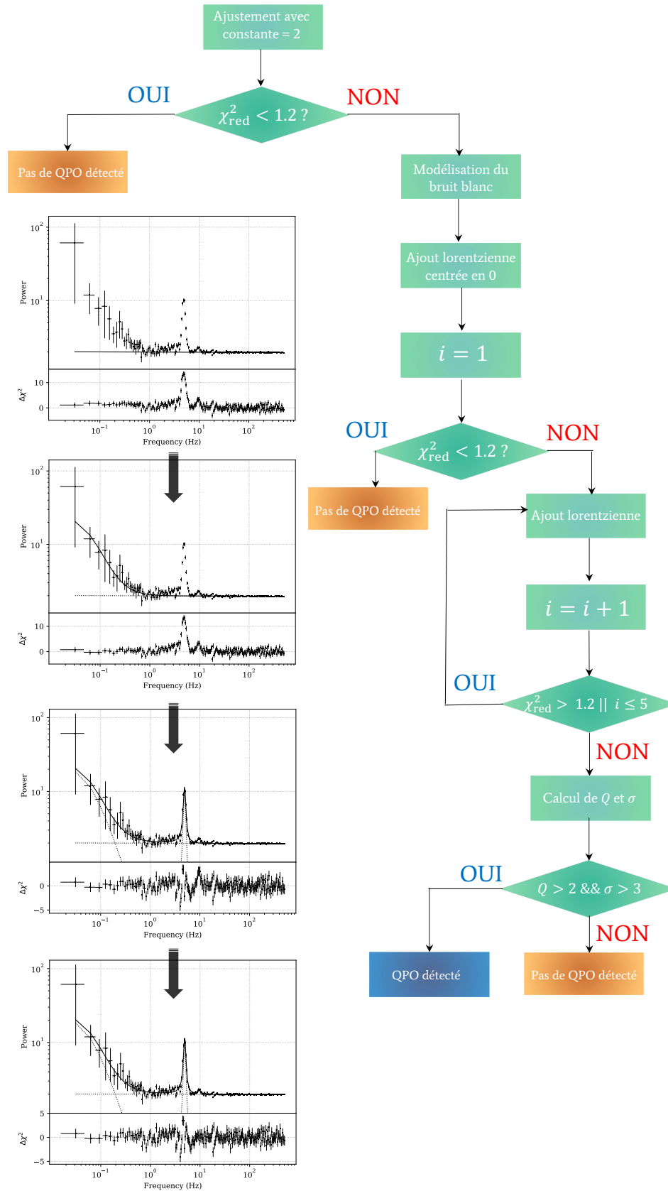
Figure 5.5 – Logigramme de la procédure permettant de détecter automatiquement des QPOs dans les spectres de puissance.
