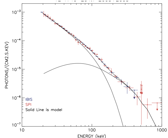
(b) Queue de haute énergie de 1E 1740.7-2942 observée avec INTEGRAL au printemps 2003. Le spectre est ajusté par deux modèles de Comptonisation thermique; l'un pour ajusté la Comptonisation inverse des photons du disque issus de la couronne, l'autre est utilisé pour ajuster l'excès à haute énergie (Bouchet et al., 2009)
