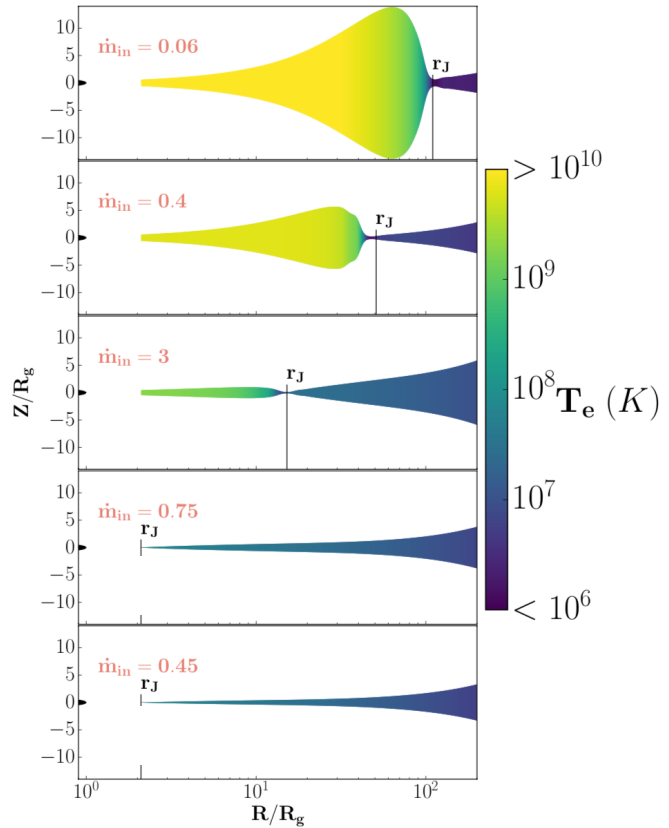
(c) Différentes configurations du disque hybride en fonction des paramètres r_{\text{J}} et \dot{m}_{\text{in}} . L’échelle de couleurs indique la température des électrons en Kelvin.
