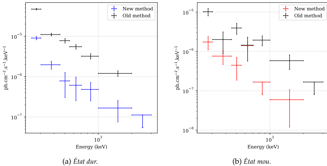
Figure 3.7 – Comparaison des spectres du mode Compton en utilisant l'ancienne méthode et la nouvelle méthode de soustraction des faux événements.
