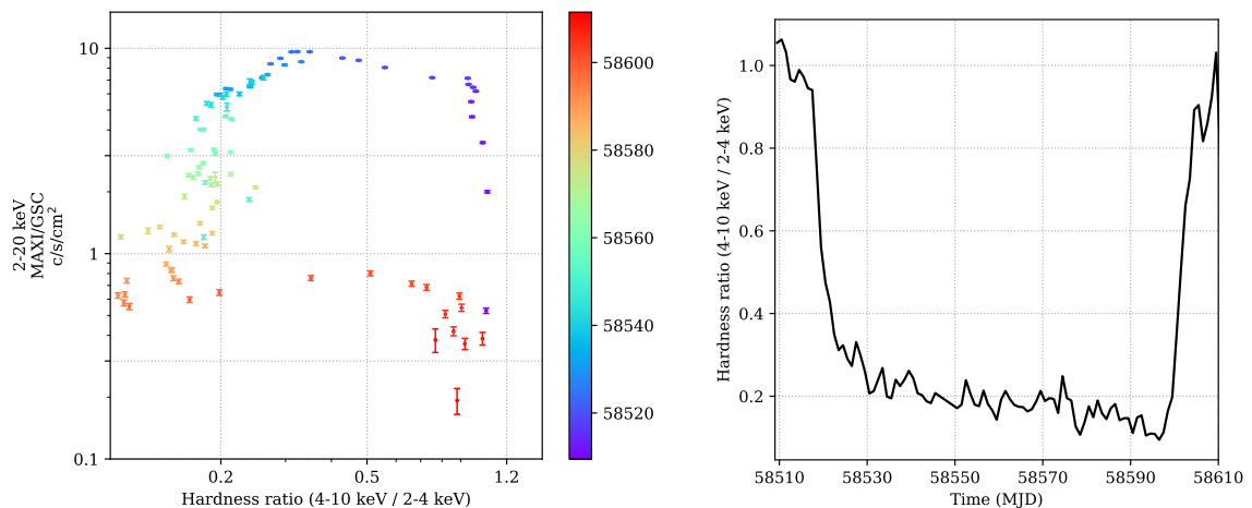
Figure 4.2 – HID de MAXI J1348–630. La carte de couleur retrace l'évolution temporelle en MJD.
