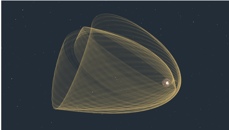
Figure 3.4 – Orbites d'INTEGRAL effectuées entre octobre 2002 et octobre 2017. Credits : ESA.
