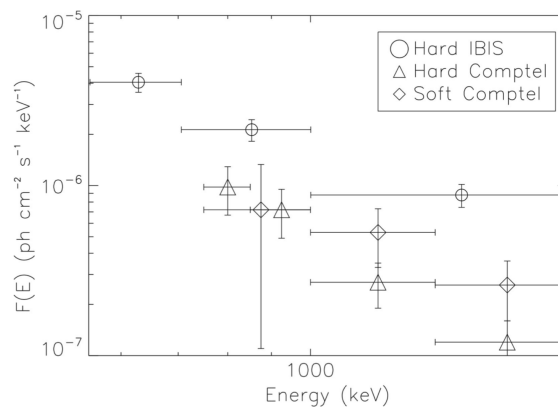
Figure 3.6 – Comparaison du spectre dur issu du mode Compton d'IBIS (cercles) avec les spectres dur et mou obtenu avec le télescope COMPTEL (triangle et losanges) ( Rodriguez et al., 2015b ).
