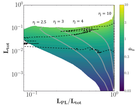
(b) L’échelle de couleurs indique l’évolution du taux d’accrétion et les contours indiquent différentes valeurs du rayon de transition r_{\text{J}} .
