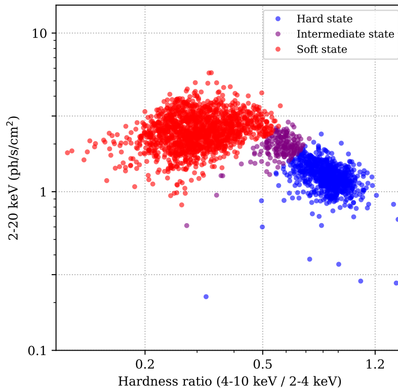
Figure 6.1 – HID de Cyg X-1 obtenu en utilisant les données de MAXI/GSC.
