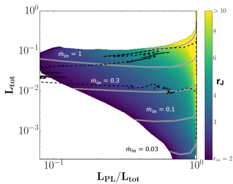
(a) L’échelle de couleurs indique l’évolution du rayon de transition r_{\text{J}} et les contours indiquent différentes valeurs du taux d’accrétion \dot{m}_{\text{in}} .
