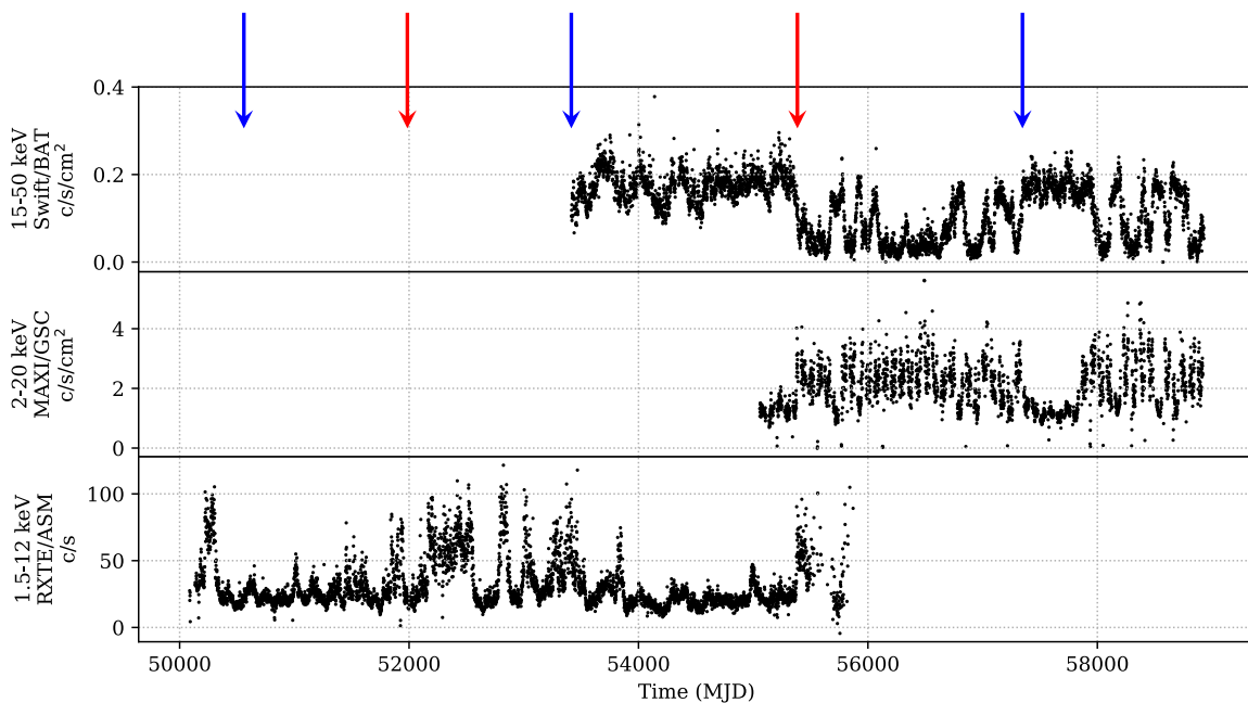
Figure 6.6 – Courbes de lumière Swift /BAT, MAXI /GSC, RXTE /ASM de Cyg X-1.
