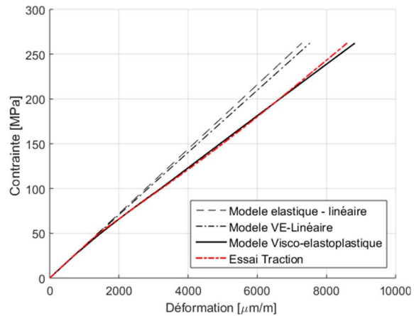
Figure 5.13 : Modélisation d'un essai de traction jusqu'à la rupture
