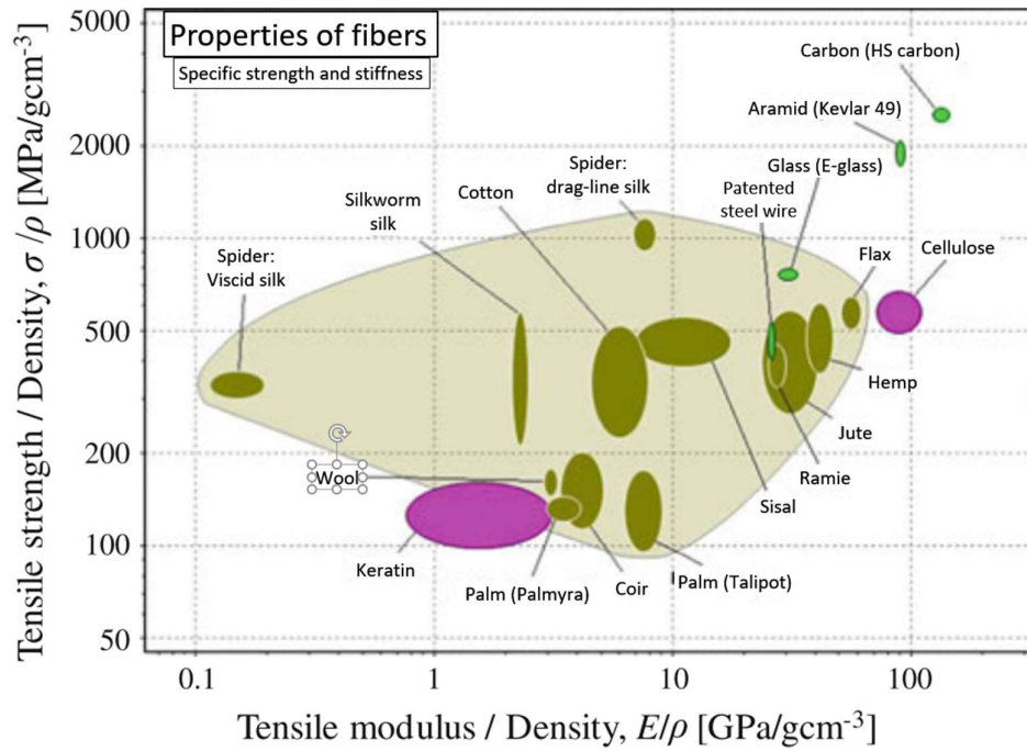
Figure 1.2: Diagramme d'Ashby des fibres de renfort [19]
