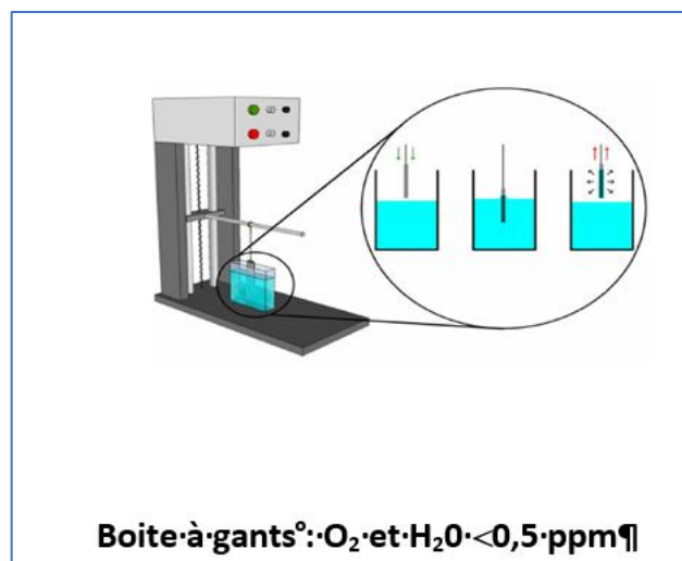
Figure 32: représentation d'un dip-coater
