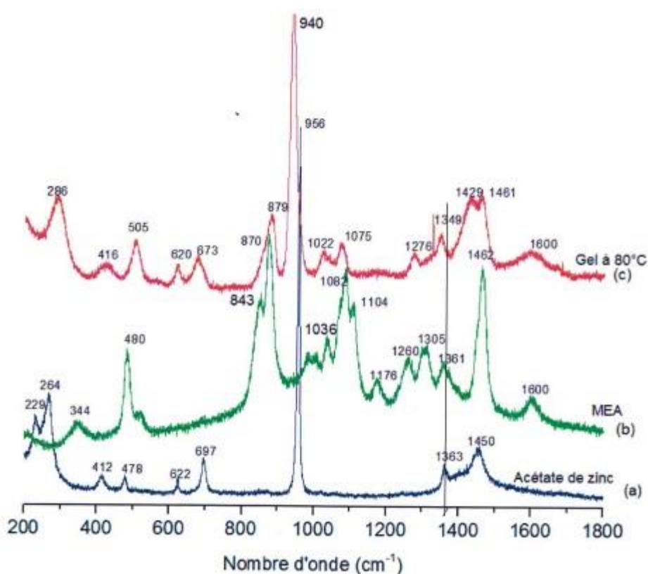
Figure 47 : Spectre Raman dans le domaine 200-1800\text{ cm}^{-1} , (a) Acétate de zinc à l'état solide, (b) MEA, (c) Gel (mélange de a et b) traité à 80^\circ C pendant 1 heure
