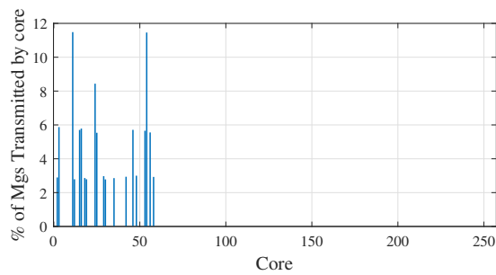
(g) SPARSE
