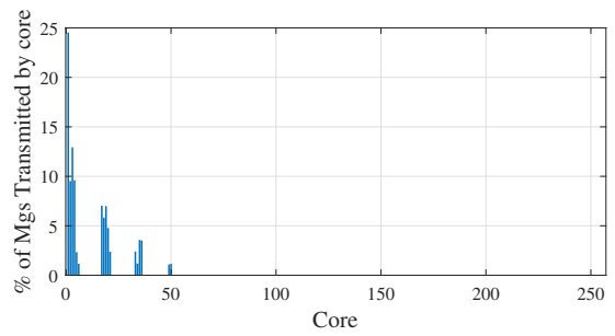
(d) ROBOT
