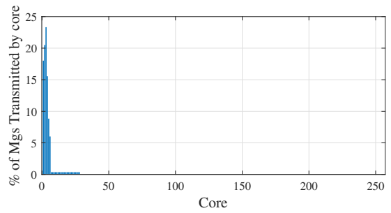
(f) RS-32_28_8_enc
