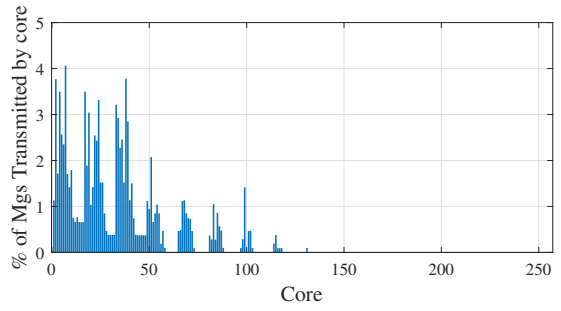
(b) FPPPP
