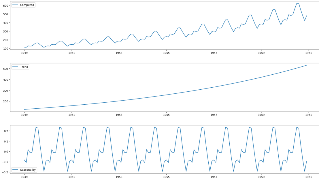
FIGURE 2.1 – Exemple d’une décomposition du phénomène cyclique et de la tendance sur le jeu de données Air Passengers.
