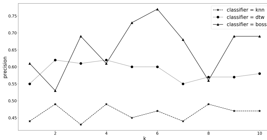
FIGURE 4.5 – Précision obtenue par les classificateurs fuzzy k-NN, F-DTW et F-BOSS en fonction du nombre de voisins k avec la stratégie 3 et \mu = 0,3 sur le jeu de données WormsTwoClass.
