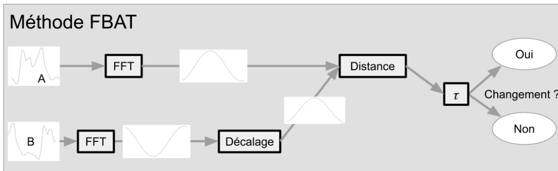
FIGURE 3.2 – Schéma global de la méthode FBAT.
