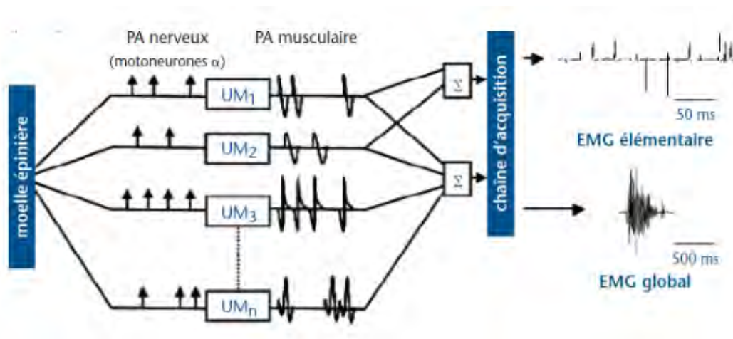
Figure 12 : correspondance physiologique du signal électromyographique. Les motoneurones alpha issus de la moëlle épinière créent des potentiels d'action « nerveux », qui en retour créent des potentiels d'action « musculaires » au niveau de l'unité motrice. La sommation du signal enregistré sur quelques unités motrices (méthode par électrode-aiguille) donne un signal EMG « élémentaire », alors que la sommation du signal créé par un plus grand nombre d'unités motrices (méthode « EMG de surface ») donne un signal EMG « global ». (Adapté de Turpin, 2012).
