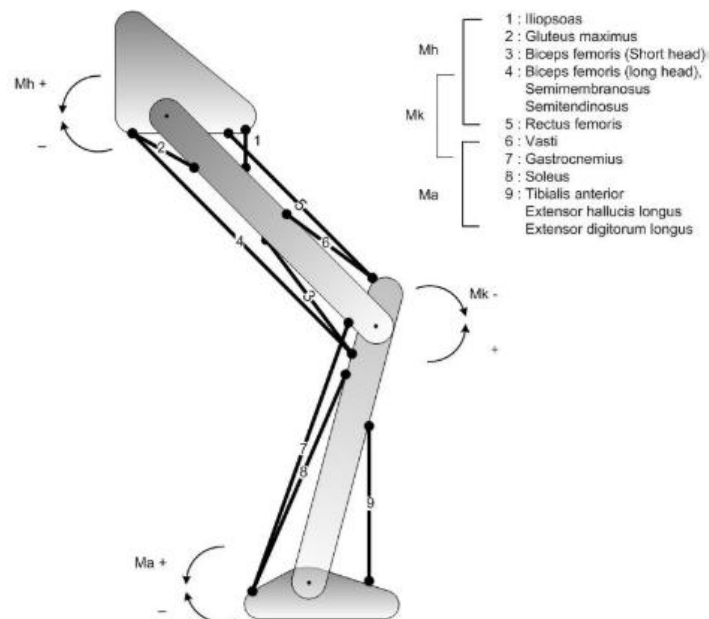
Figure 10 : représentation schématique des principaux muscles actionneurs du membre inférieur. Ma , Mk et Mh représentent les moments résultants au niveau de la cheville, du genou et de la hanche, respectivement. (Adapté de Poirier, 2009).
