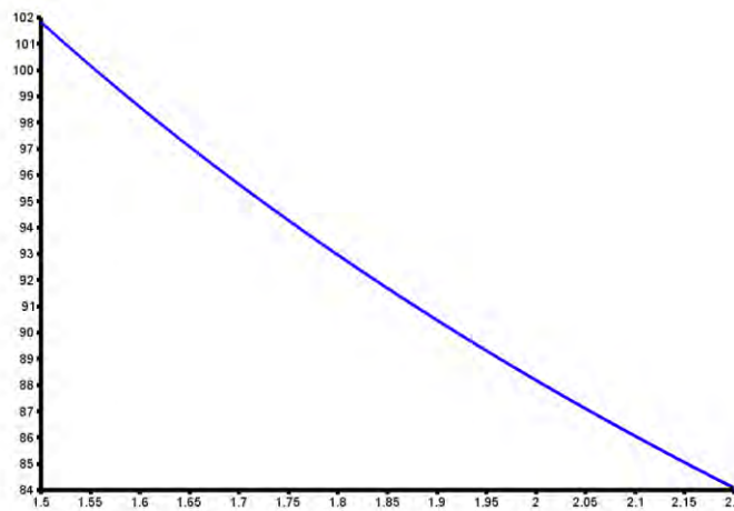
Figure 31 : fréquences de pédalage similaires exprimées en RPM (Rotations Par Minute) exprimées en fonction de l'anthropométrie des cyclistes.
