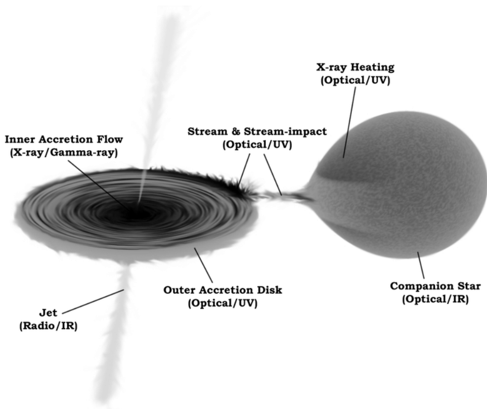
FIGURE 1.2 – Illustration schématique d’une binaire X de faible masse et du transfert de masse par débordement du lobe de Roche menant à l’émission de jets. (Hynes, 2010).
