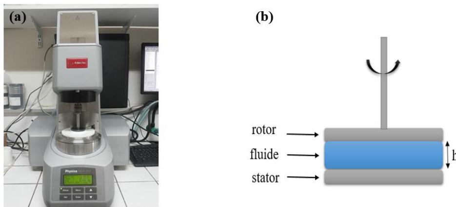
Figure II-12 : (a) Rhéomètre Anton Paar MCR 30, (b) Rhéomètre représentation géométrie plan-plan.
