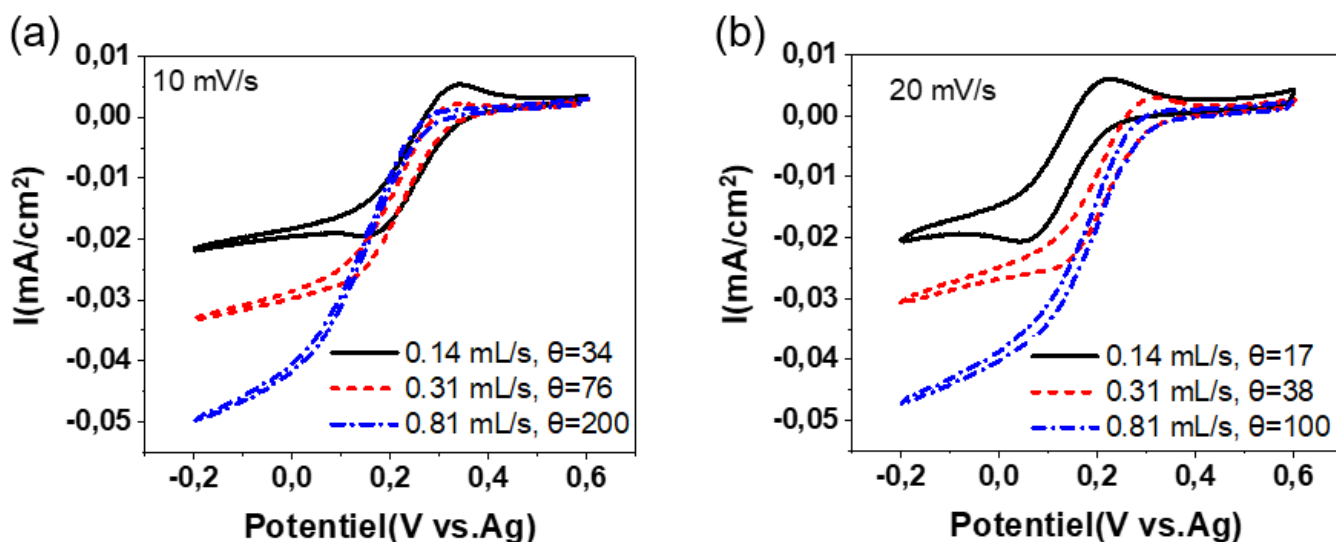
Figure IV-5 : Effet de la variation du débit d'écoulement sur le signal électrochimique avec l'utilisation de Pt comme électrode de travail à des vitesses de balayages de (a) 10 mV/s et (b) 20 mV/s.
