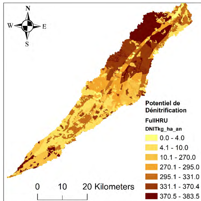
Figure 116: Cartographie du potentiel de dénitrification du bassin versant de la Save en \text{kg} \cdot \text{ha}^{-1} \cdot \text{an}^{-1} simulé en 2010,
