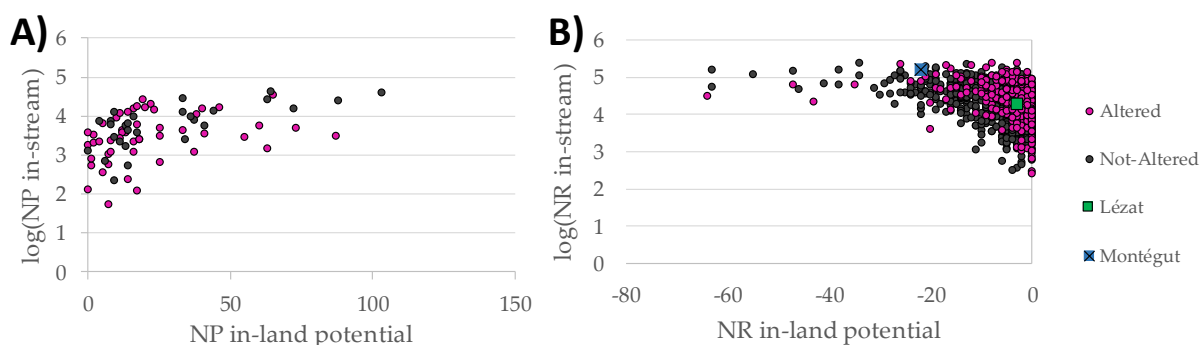
Figure 84: Corrélation entre le potentiel des bilans nets en nitrates (NNB) terrestres et le logarithme des NNB aquatiques ( \text{kgN}\cdot\text{m}^{-2}\cdot\text{yr}^{-1} ) pour (A) la fonction d'élimination des nitrates (NR avec \text{NNB}<0 ) et (B) la fonction de production des nitrates (NP avec \text{NNB}>0 ). Les carrés indiquent les sous-systèmes auxquels appartiennent les tronçons de Lézat et de Montégut mesurés dans le projet STREAMES (Chapitre 3B).
