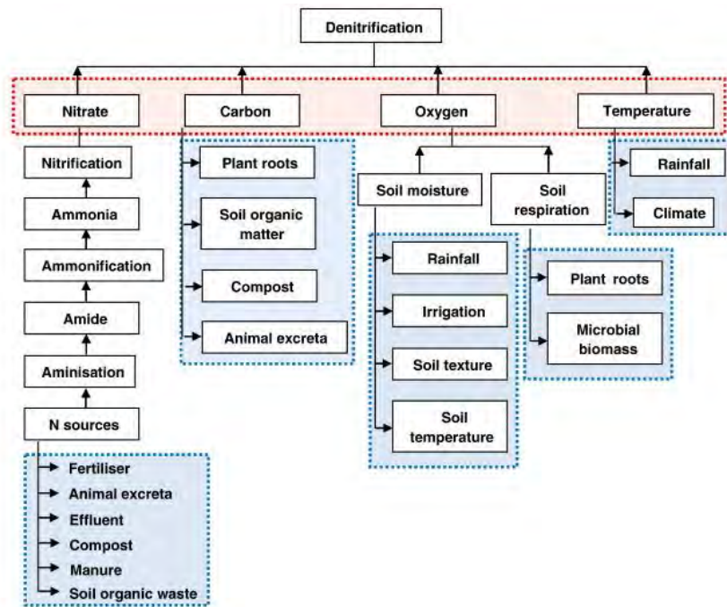
Figure 14: Facteurs influençant la dénitrification dans les sols (rouge : facteurs directs, bleus: facteurs indirects) tirés de Saggari et al. (2013).
