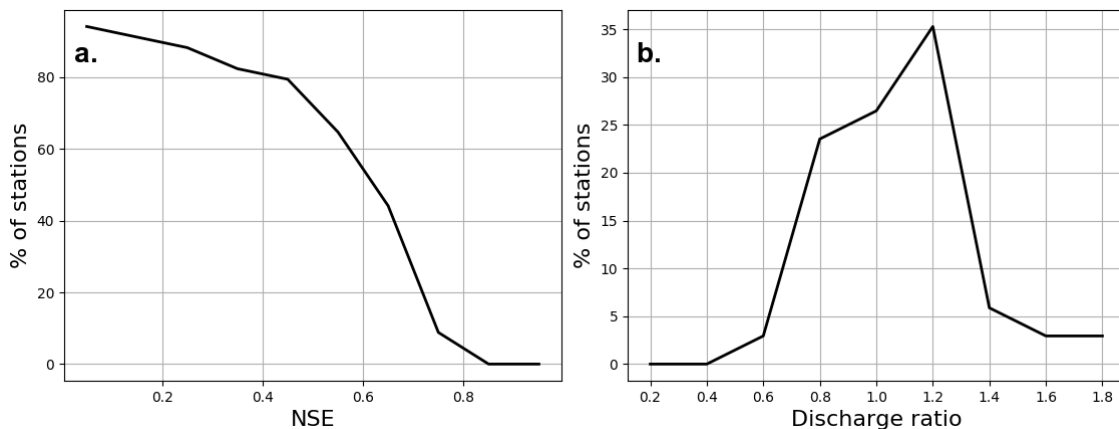
Figure 103: (a) Pourcentage de pixel de SIM pour chaque station de validation en fonction des performances de Nash-Sutcliff Efficiency (NSE) et (b) le rapport de débit au 34 stations de contrôle entre 1958 et 2016 (issus de Biancamaria et al., 2019).
