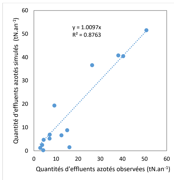
Figure 29: Comparaison entre les effluents azotés en tN.an -1 observés par les agences de l'eau (de 2000 à 2010) et celles simulées avec l'équation 37 issue des données de la base de données UWWTP—EUDB ( https://ec.europa.eu/ ).
