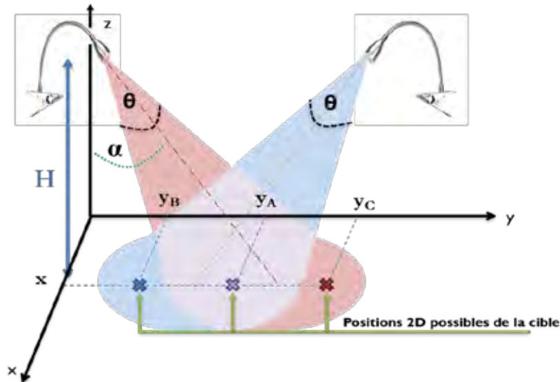
Figure 3.16- Intersection de deux faisceaux lumineux
